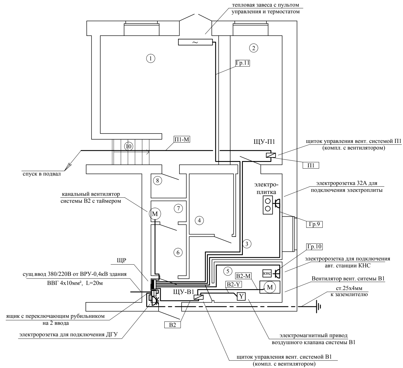
План 1 этажа М 1:100
