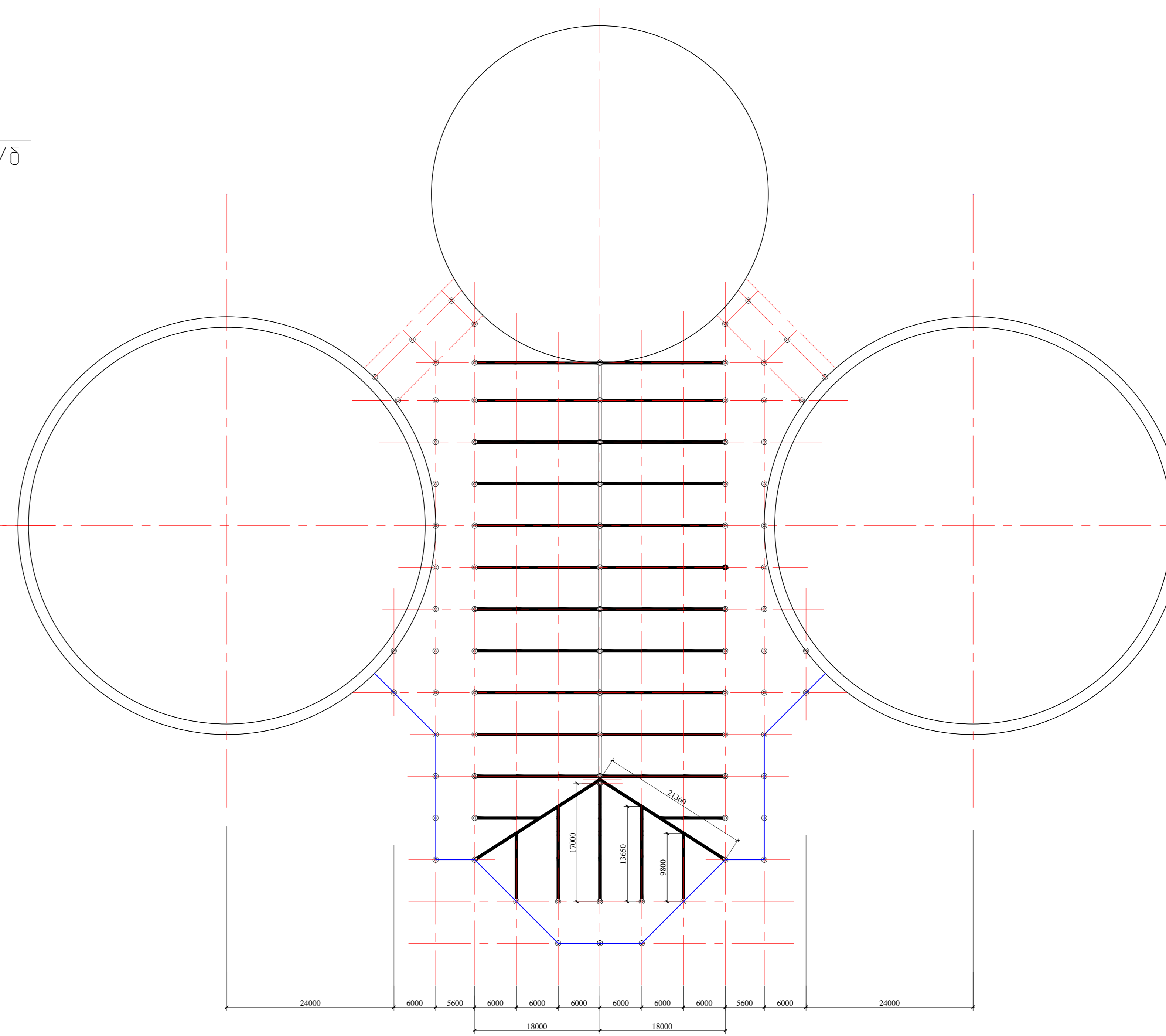
СХЕМА РАСПОЛОЖЕНИЯ ФЕРМ ПОКРЫТИЯ.
