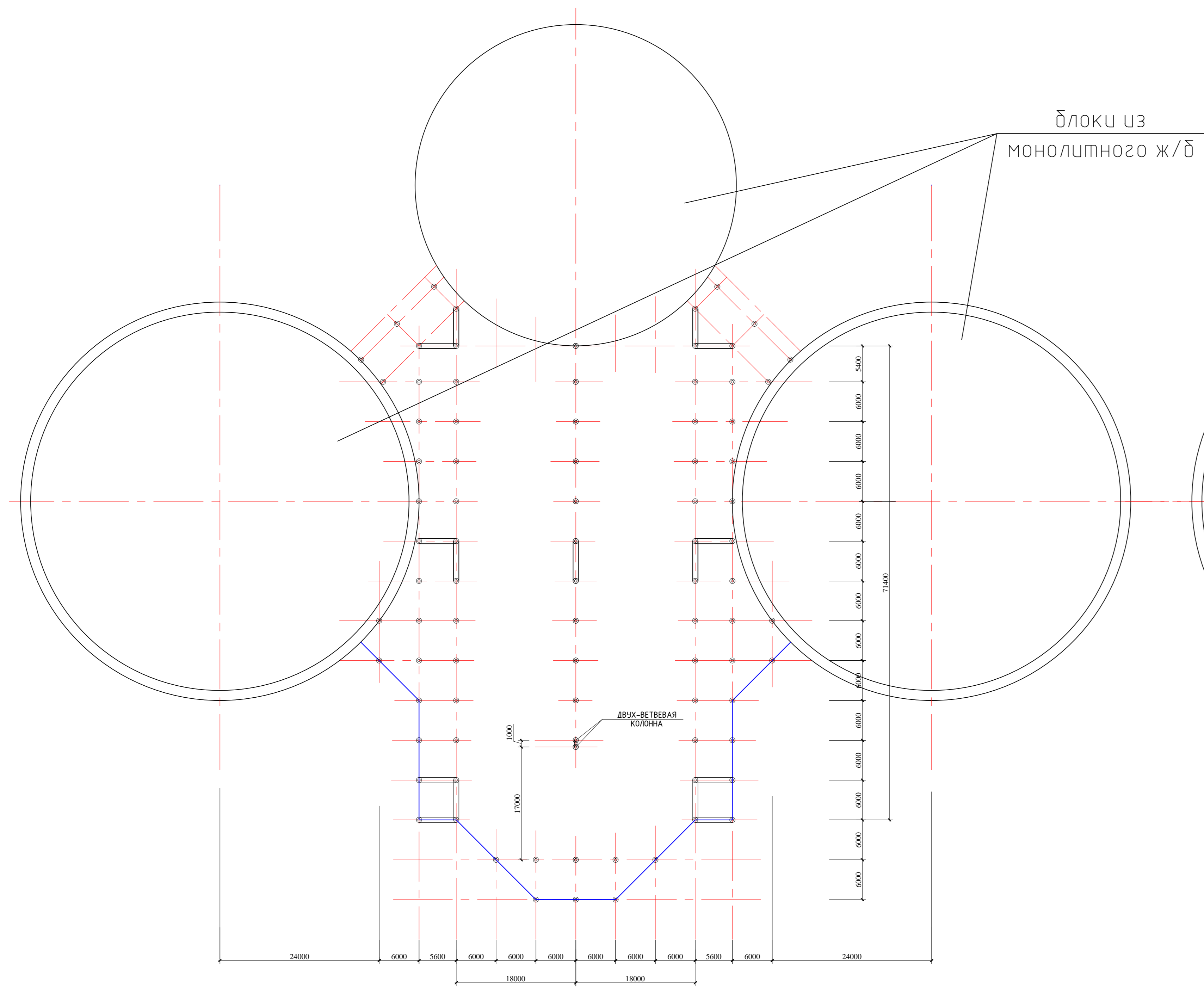
СХЕМА РАСПОЛОЖЕНИЯ КОЛОНН И ВЕРТИКАЛЬНЫХ СВЯЗЕЙ КАРКАСА.
