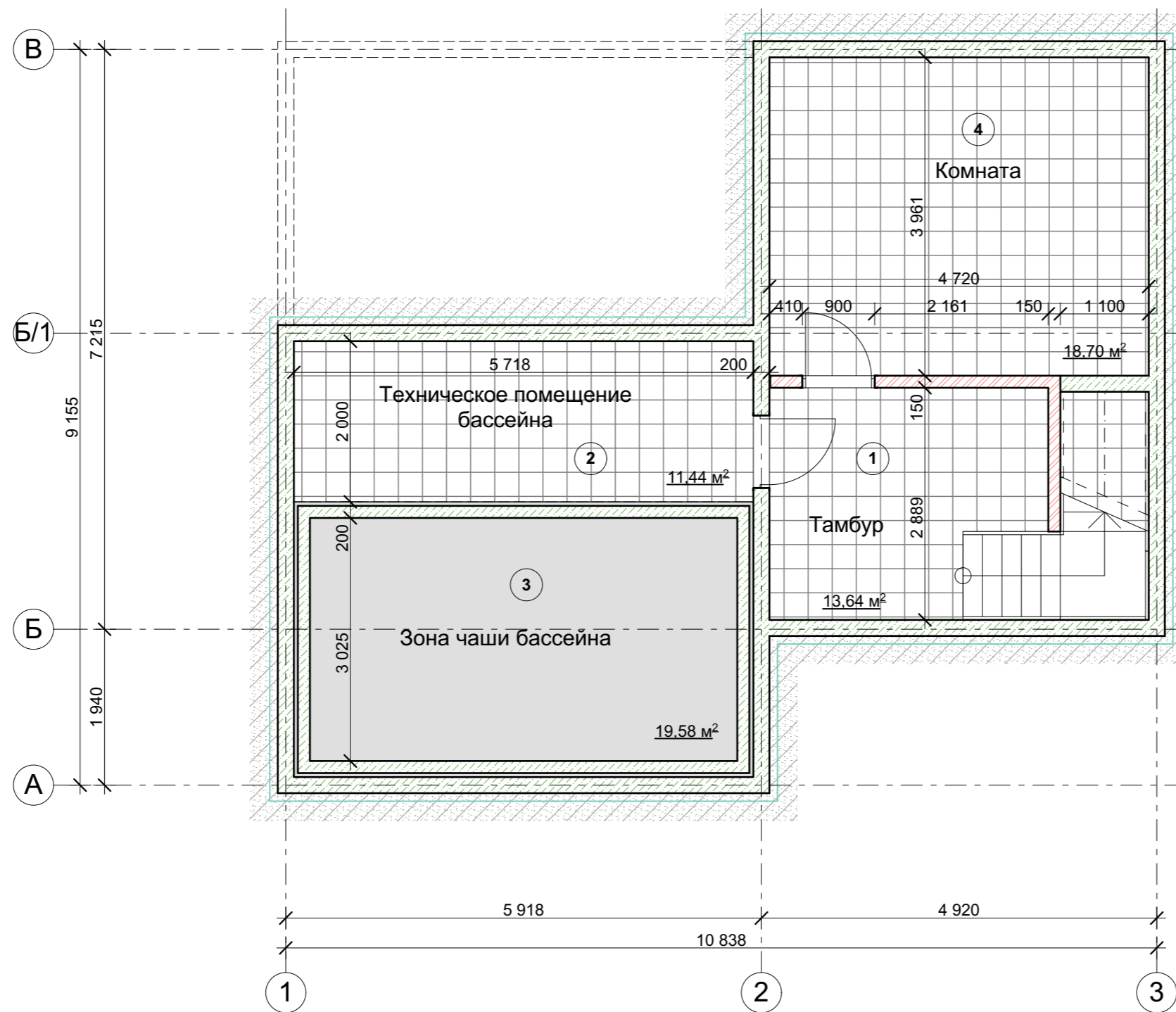
Экспликация помещений подвального этажа
