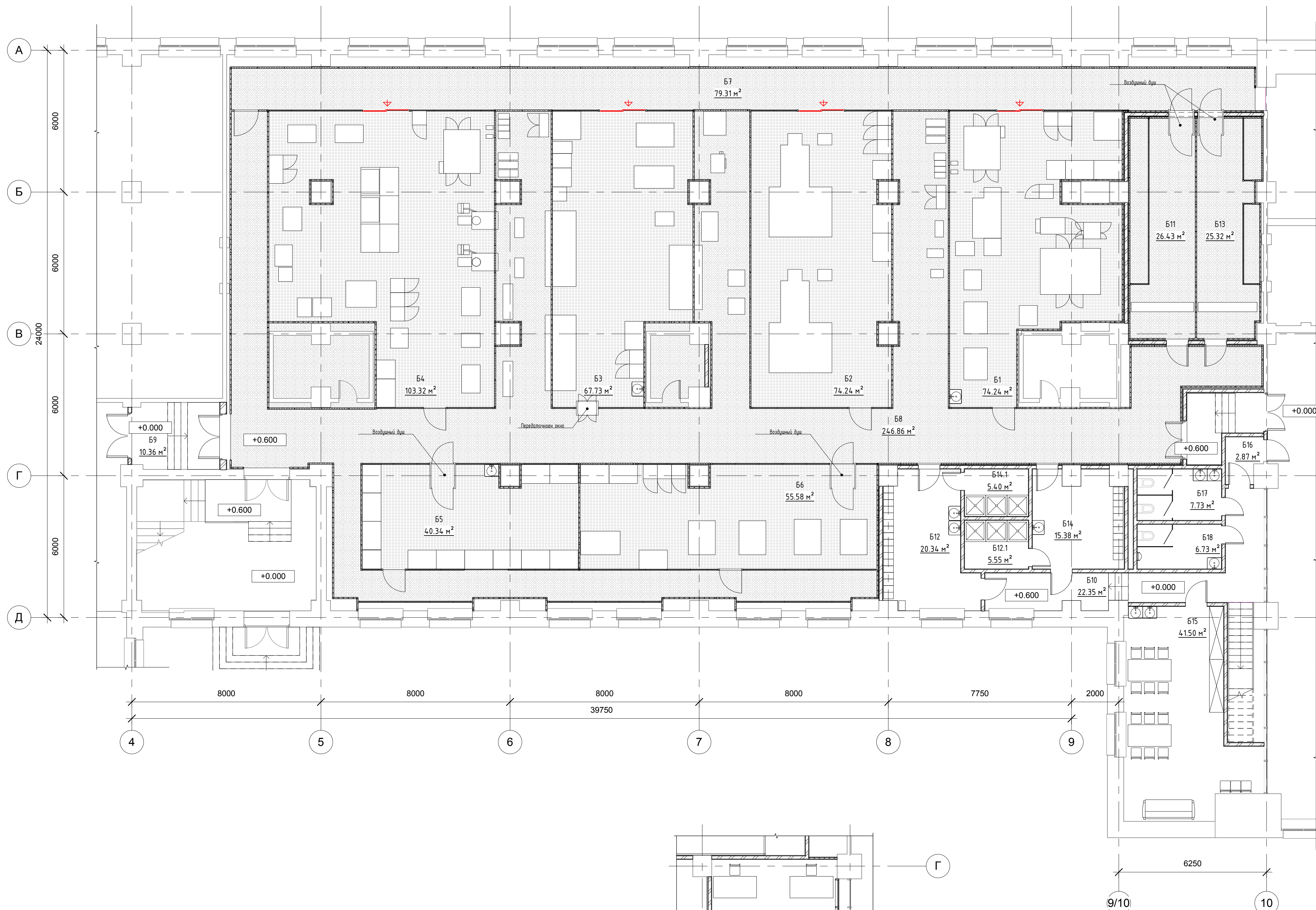
3 План антресоли 1 : 100
