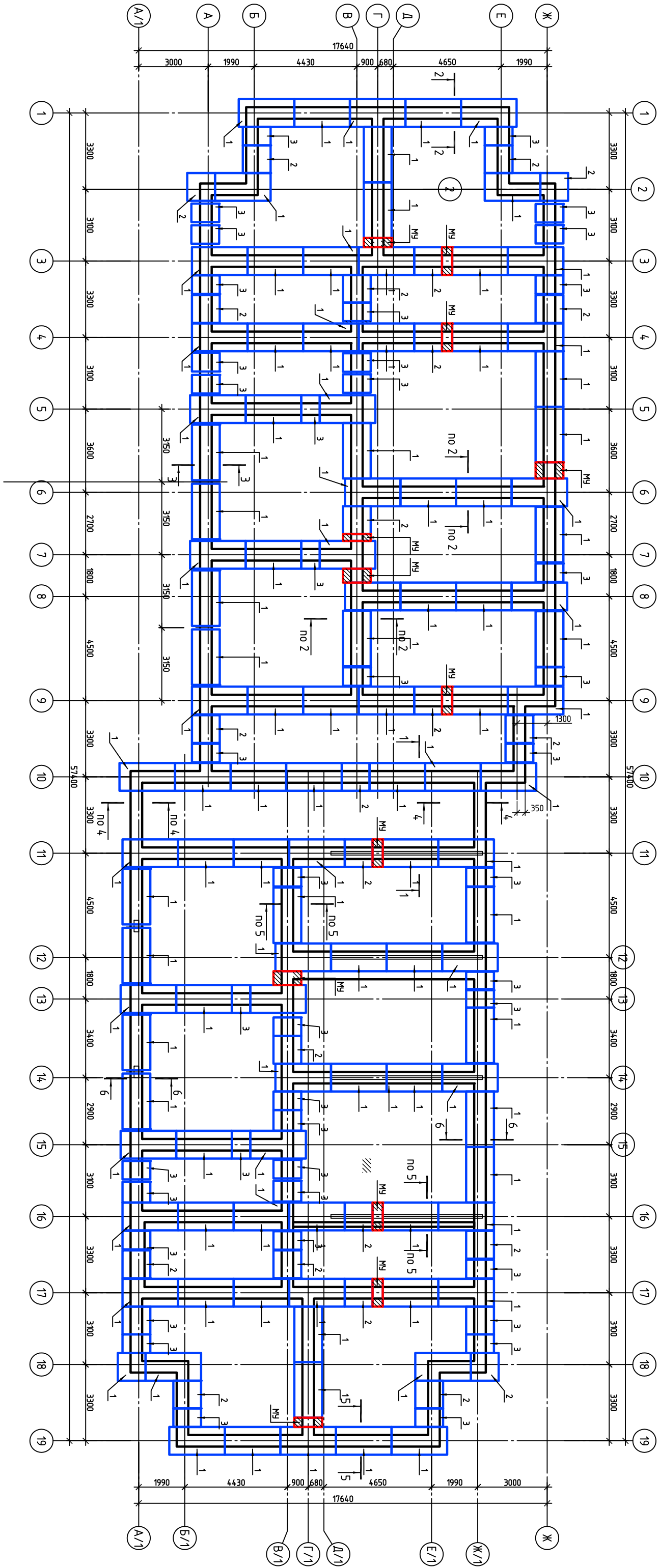
Схема расположения элементов фундаментов на отметках -2,760 (нуз), -1,560 (нуз)
