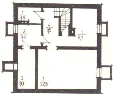
ПЛАН ПОДВАЛА
