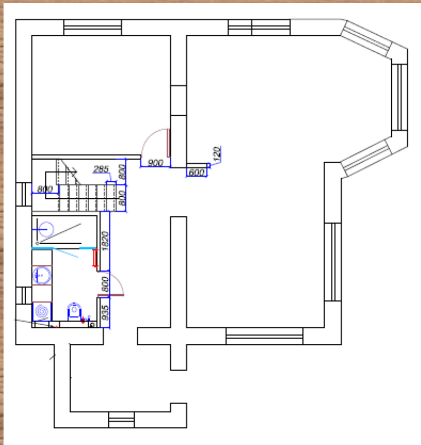
План 1го этажа 87м 2
