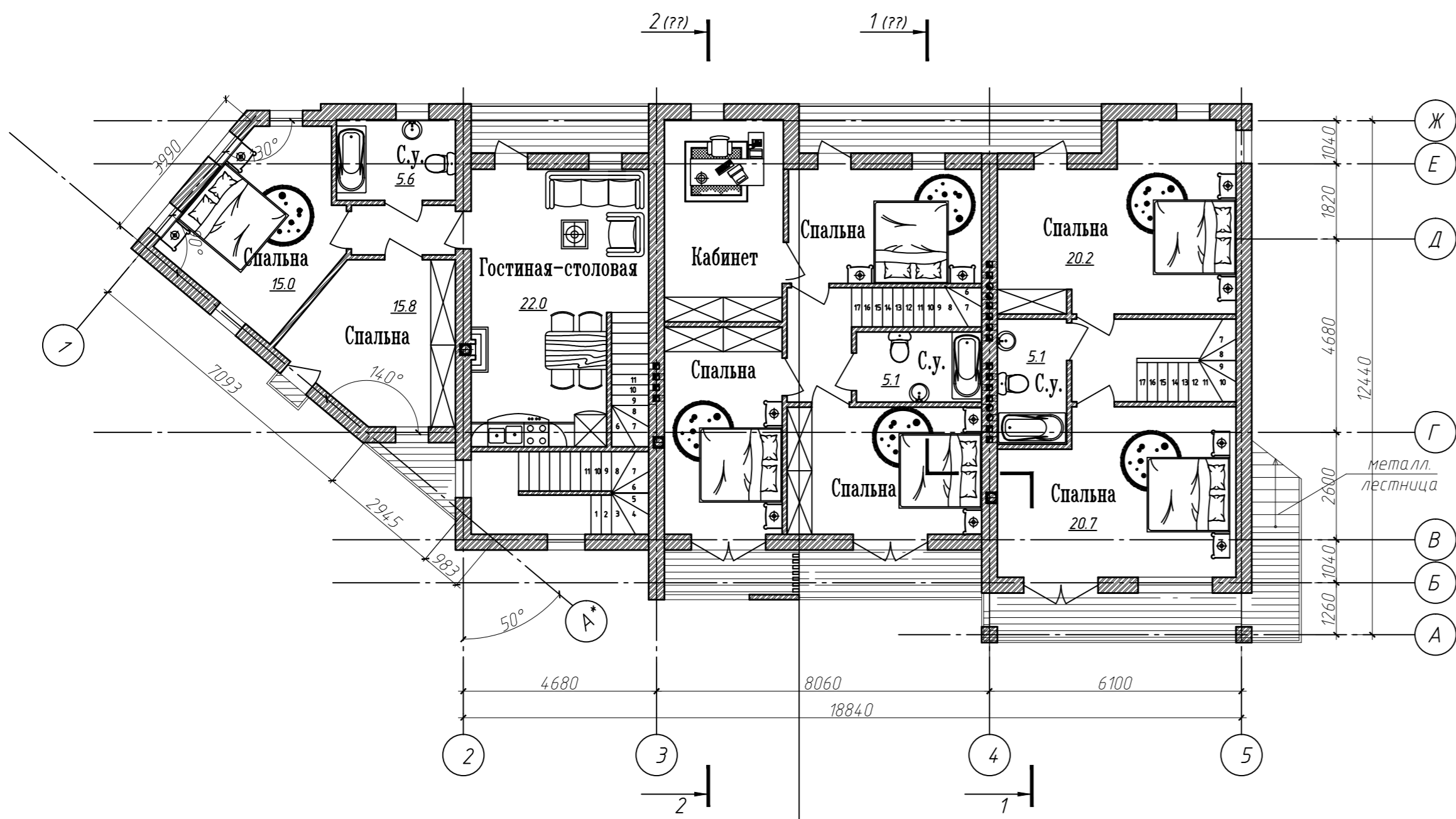
ПЛАН 2 ЭТАЖА
