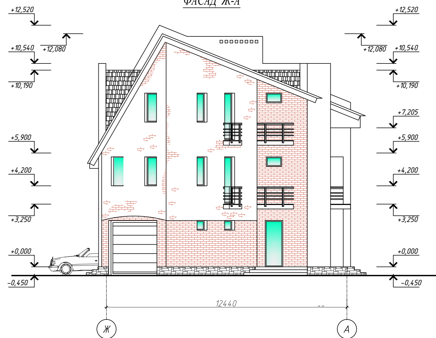
ФАСАД Ж-А
