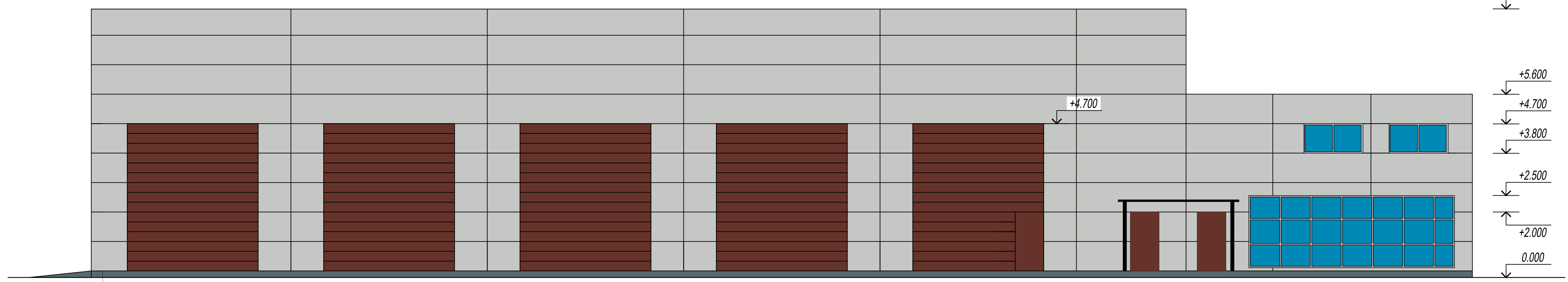
Фасад в осях 9-1 М 1:50
