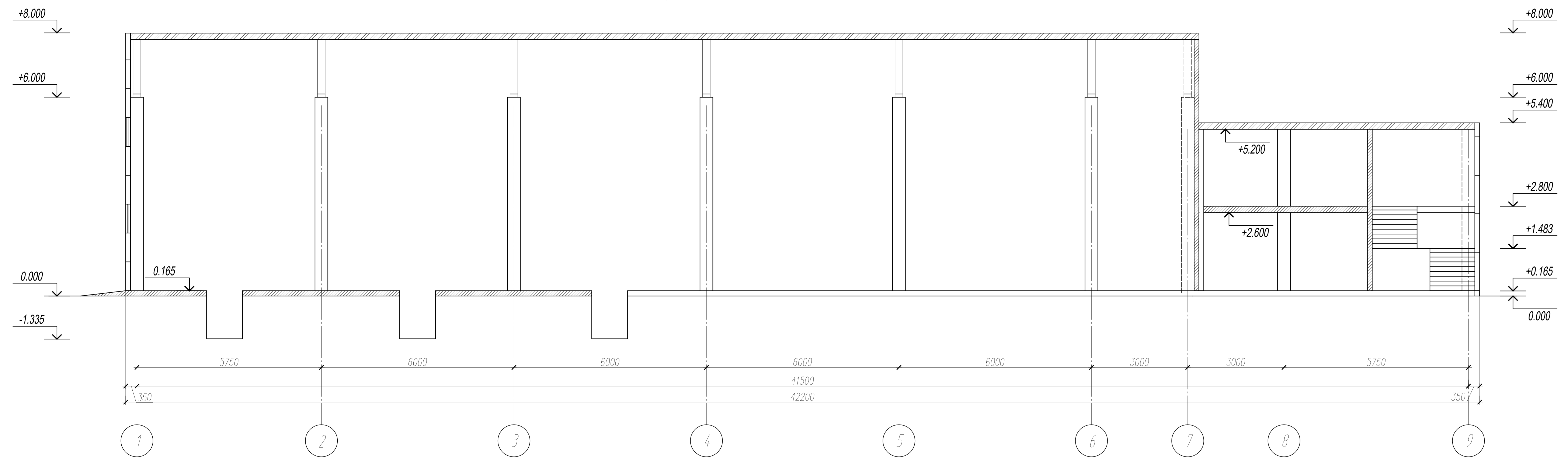
Разрез 2-2 М 1:50
