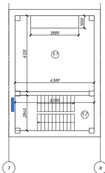
План подвала в осях 3-3с на отм. -3.500
