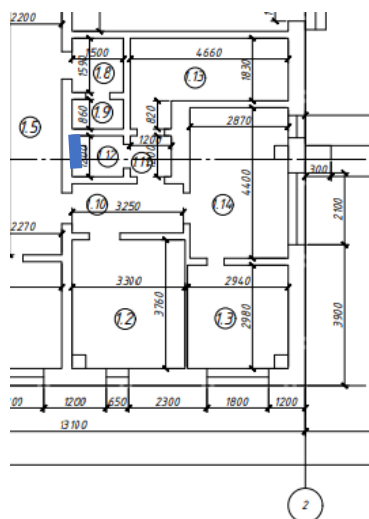
Трещины на внутренней стене здания между осями 1-2 по оси Б в пом.1.12
