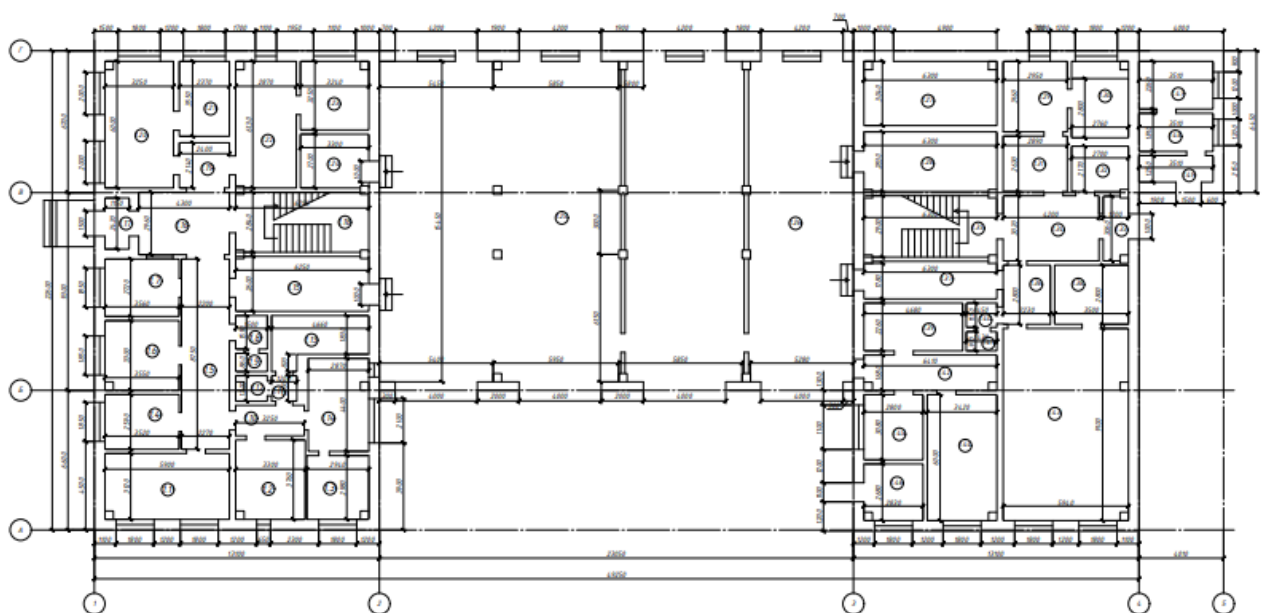
Рисунок 3.1 Схема этажа с обозначением мест испытания конструкций стен
