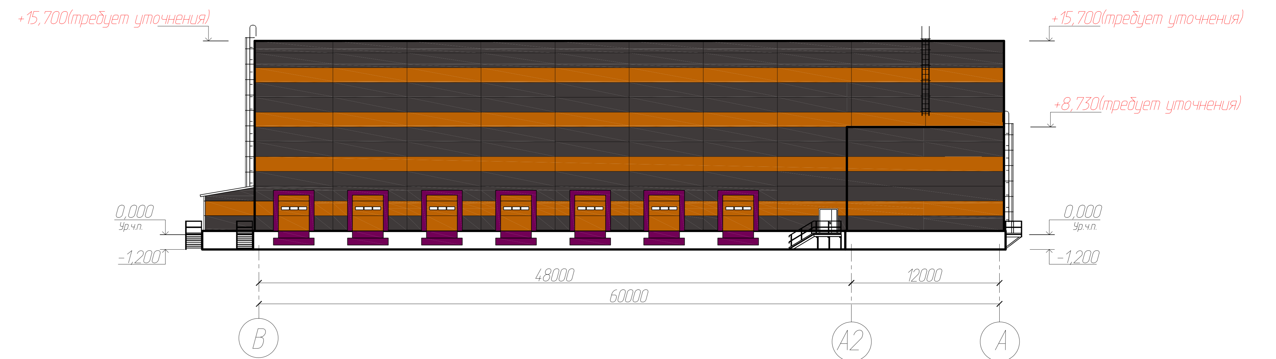
Фасад в осях В-А
