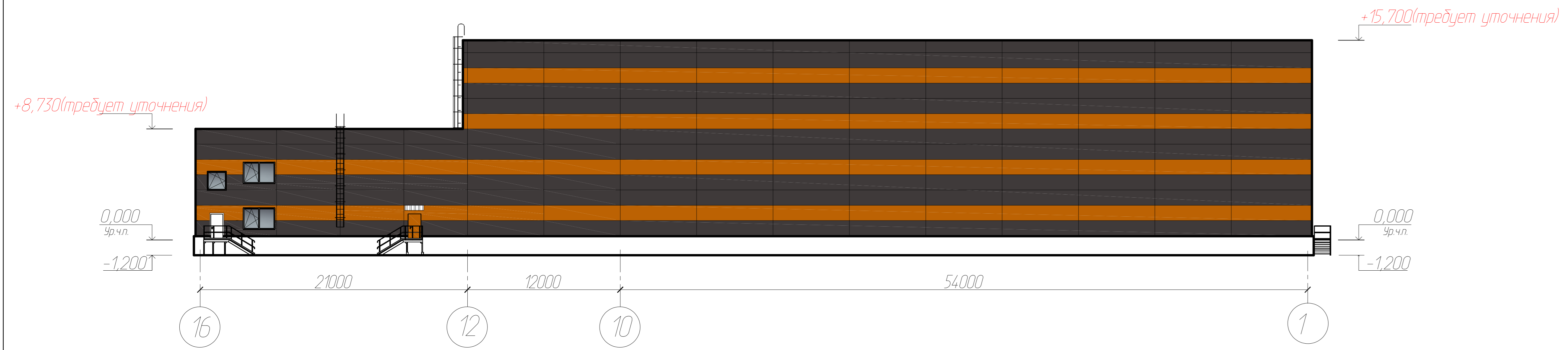
Фасад в осях 16-1
