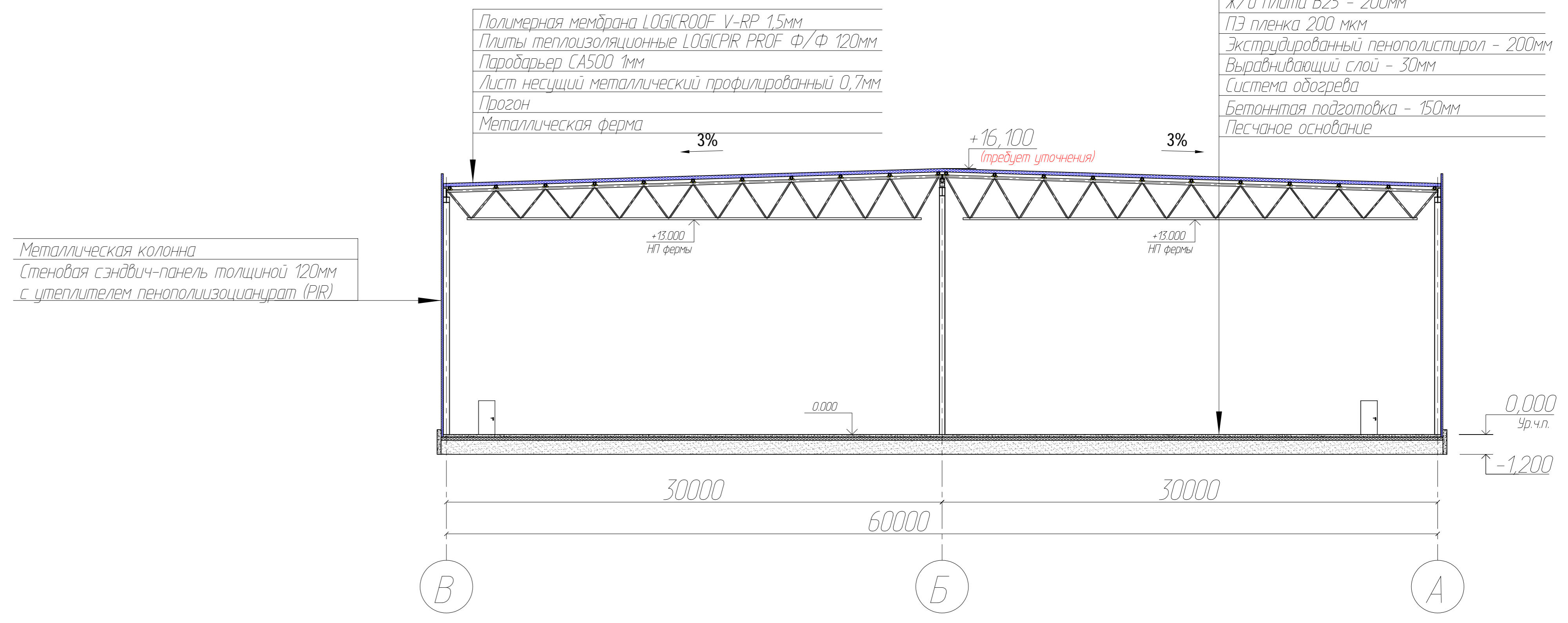
Разрез 2-2 (зона логистики)
