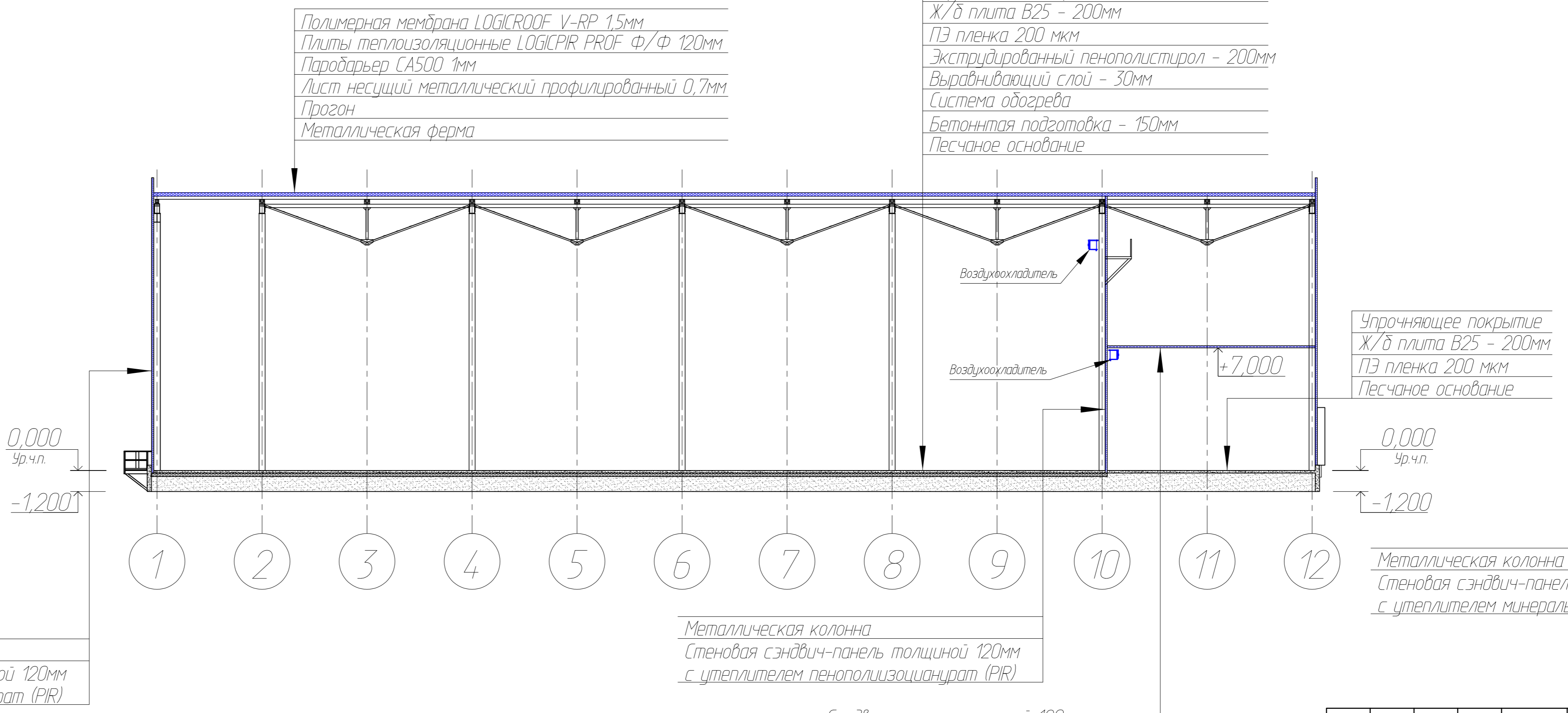
Разрез 3-3
