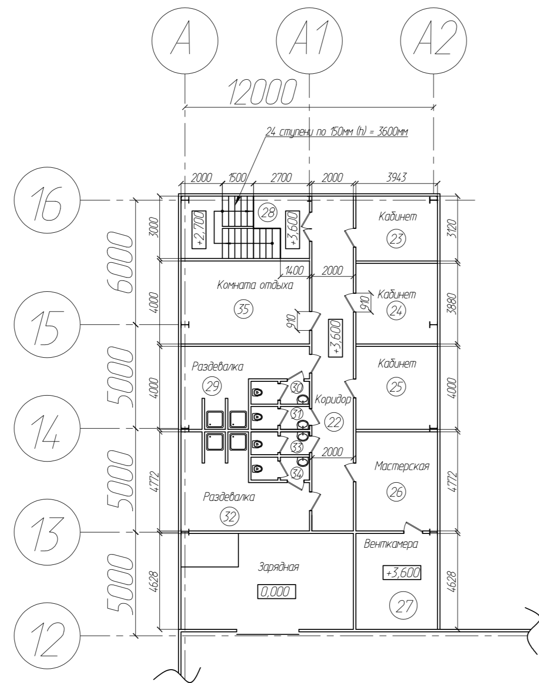
План на отм. +3,600.
