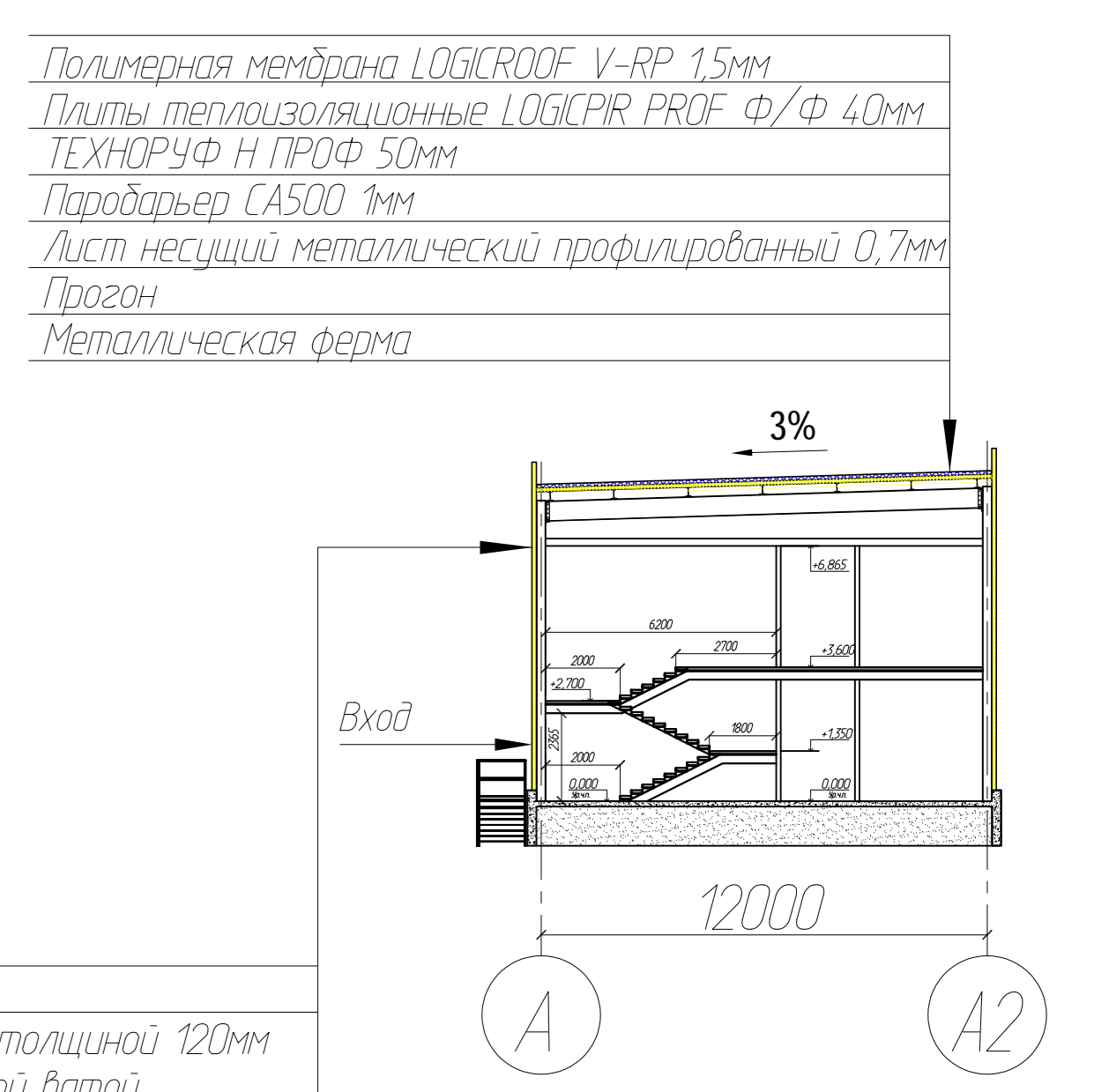
Разрез 4-4
