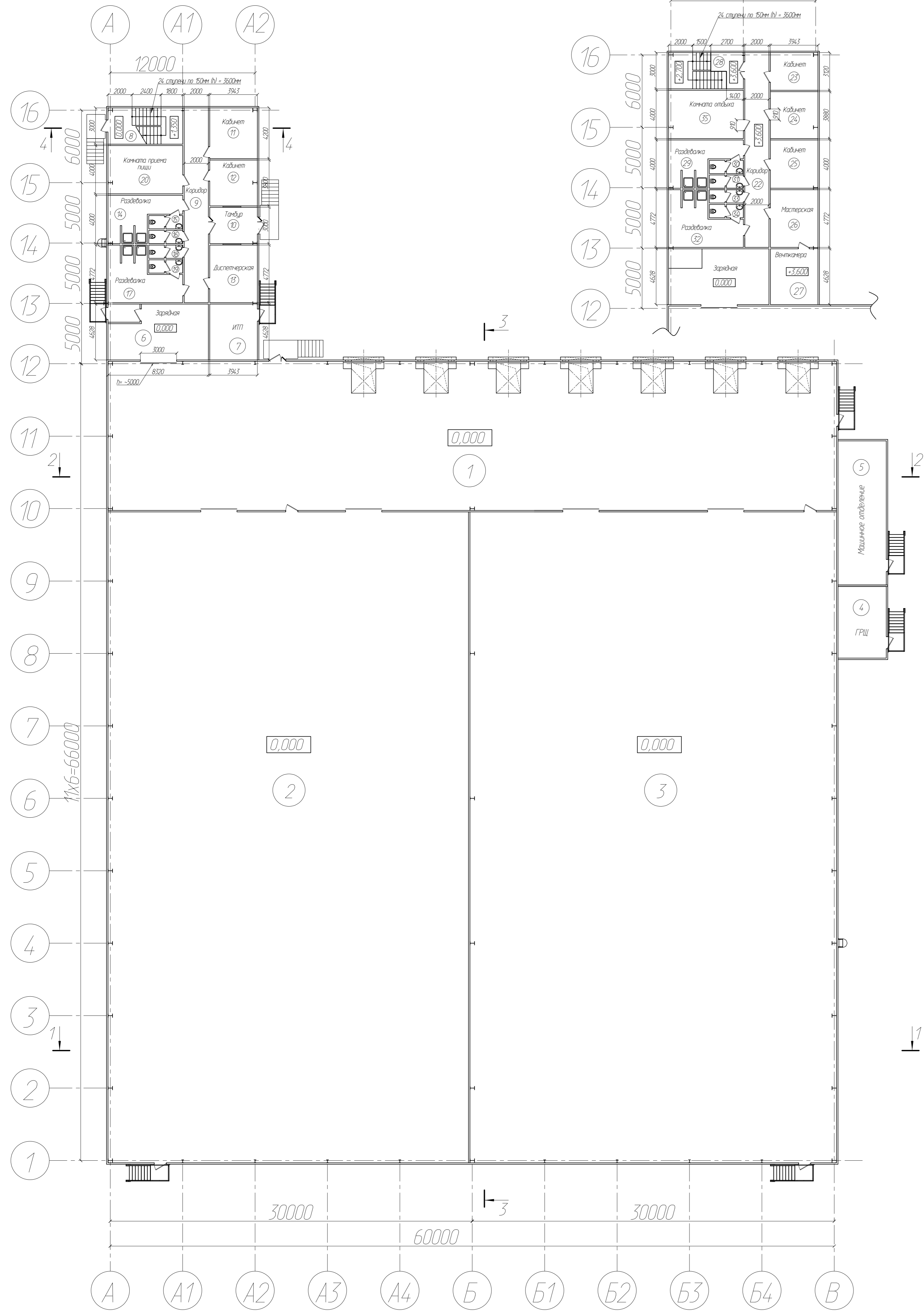
План на отм. 0,000.
