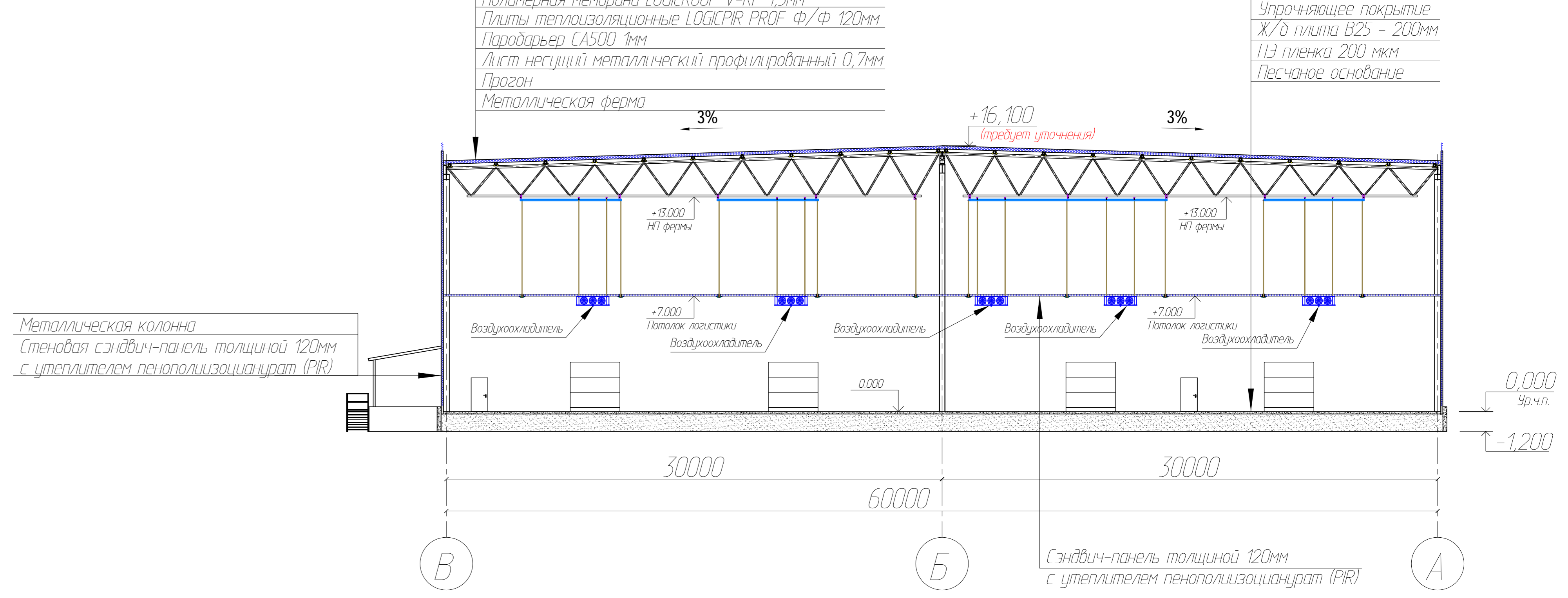
Разрез 3-3
