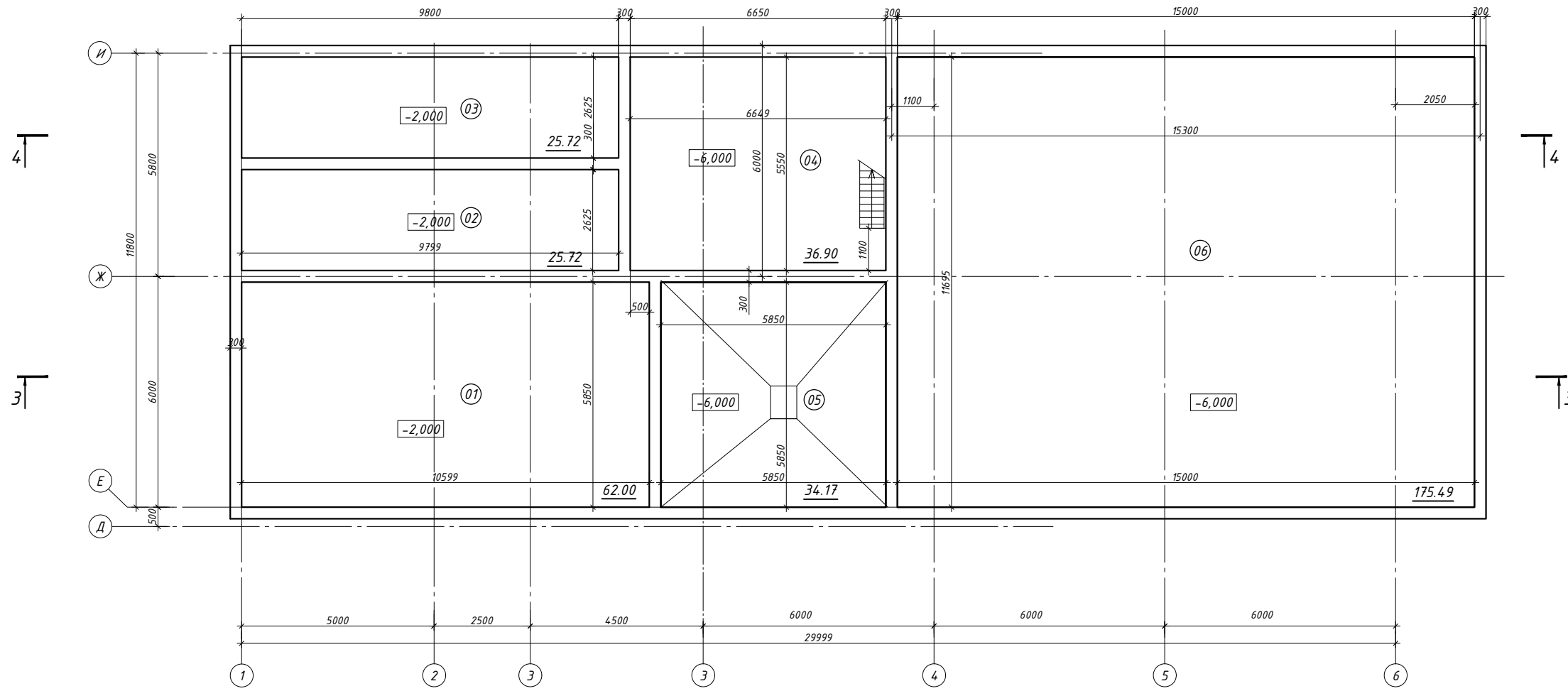
План на отм -6.000
