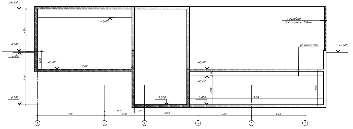
Разрез 3-3
