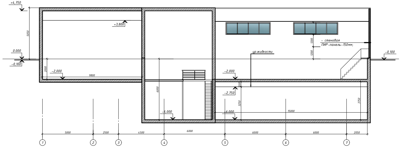
Разрез 3-3
