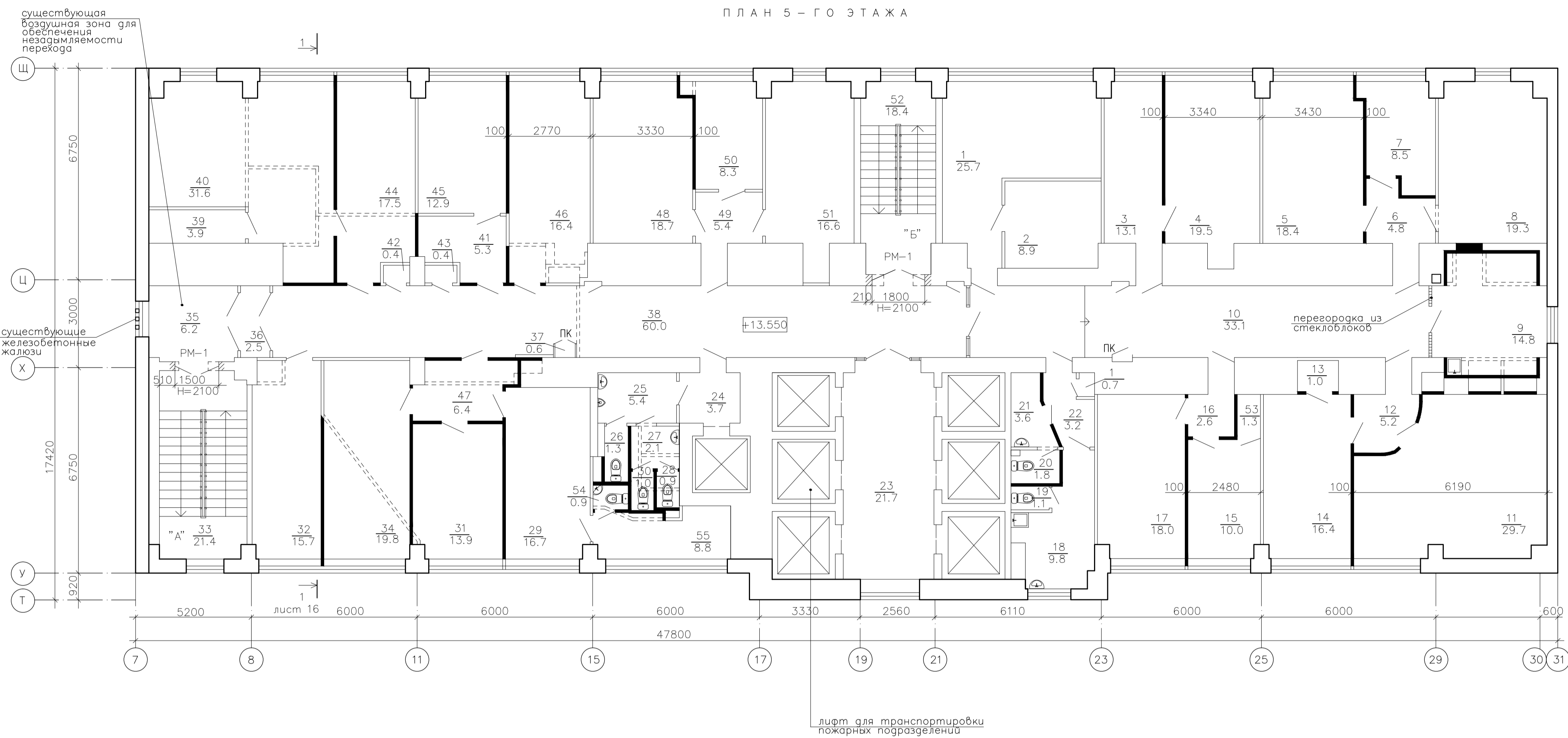
ПЛАН 5 - ГО ЭТАЖА
