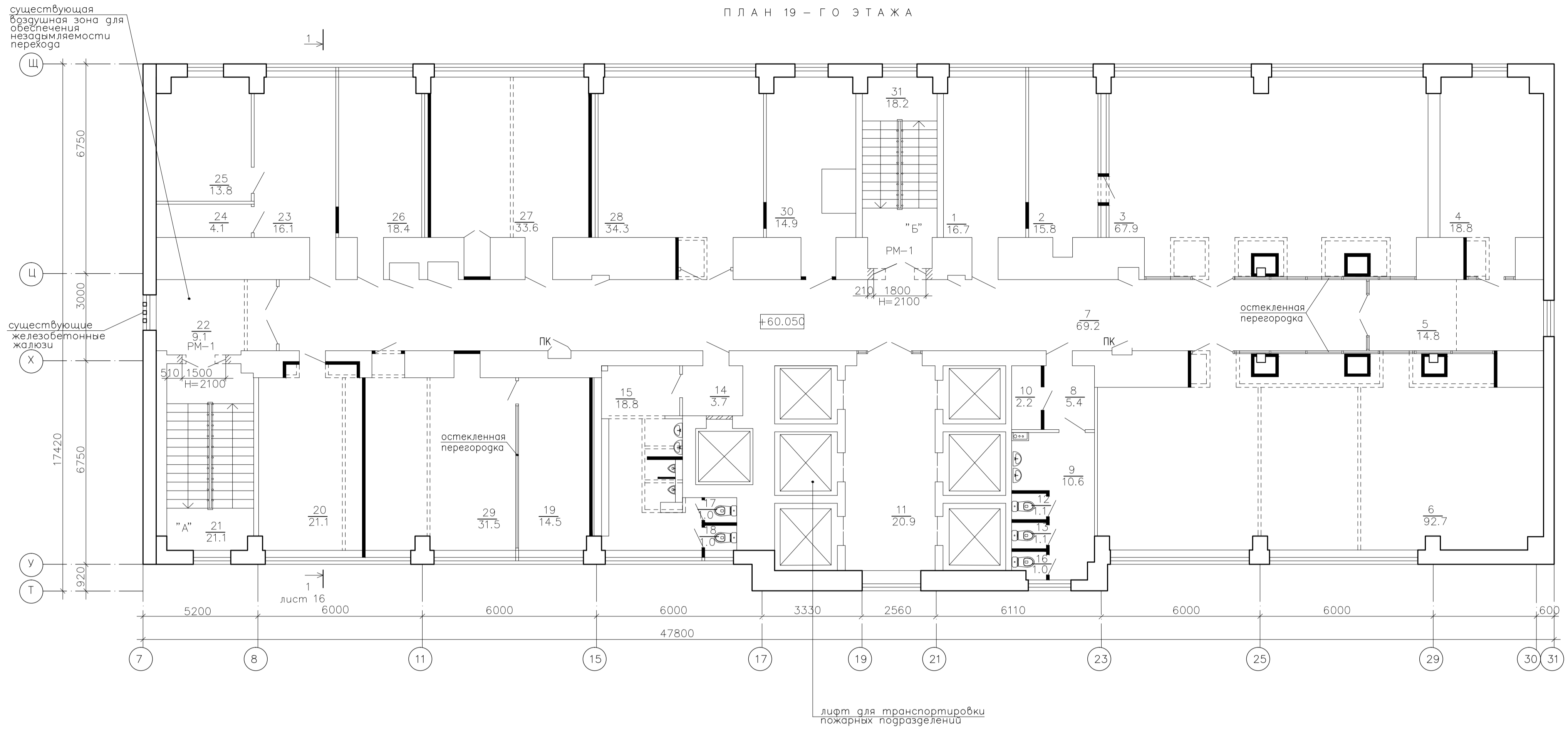
ПЛАН 19 - ГО ЭТАЖА
