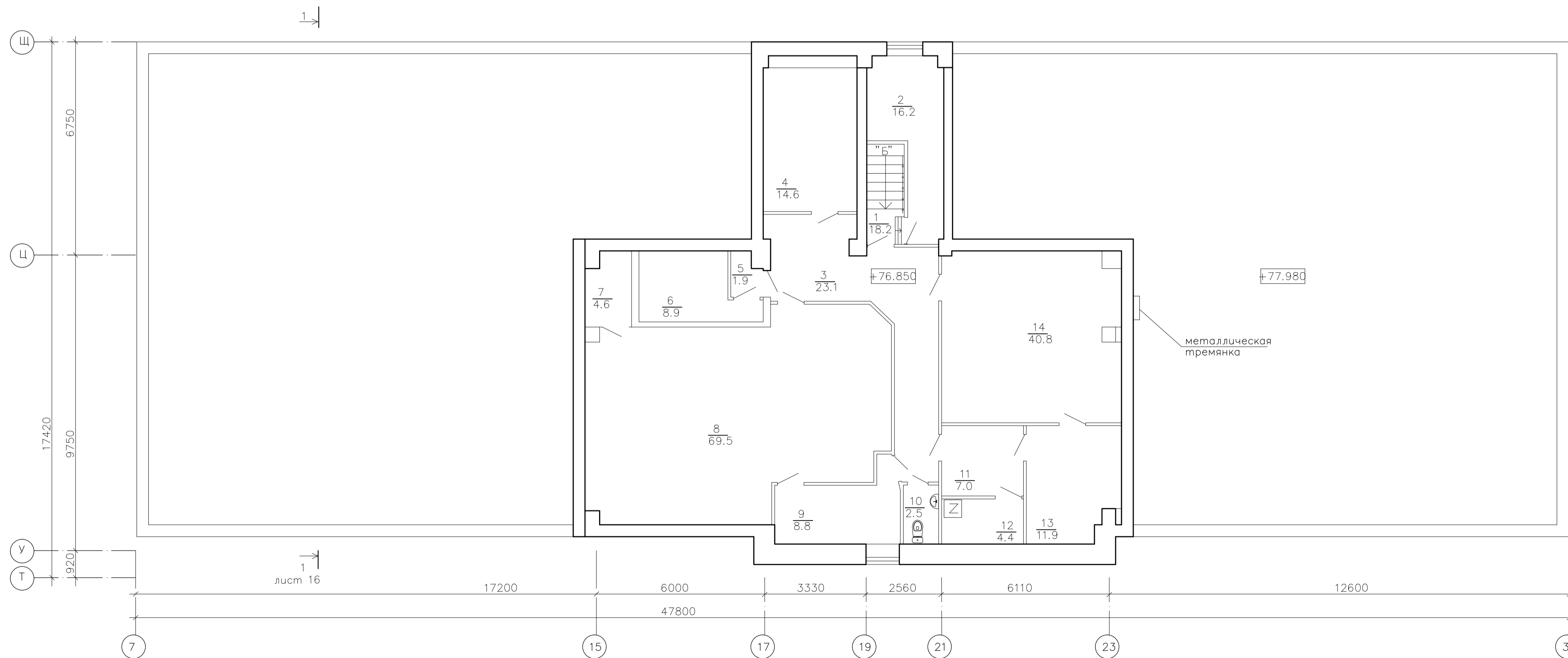
ПЛАН ТЕХНИЧЕСКОГО ЭТАЖА НА ОТМ. +76.850М
