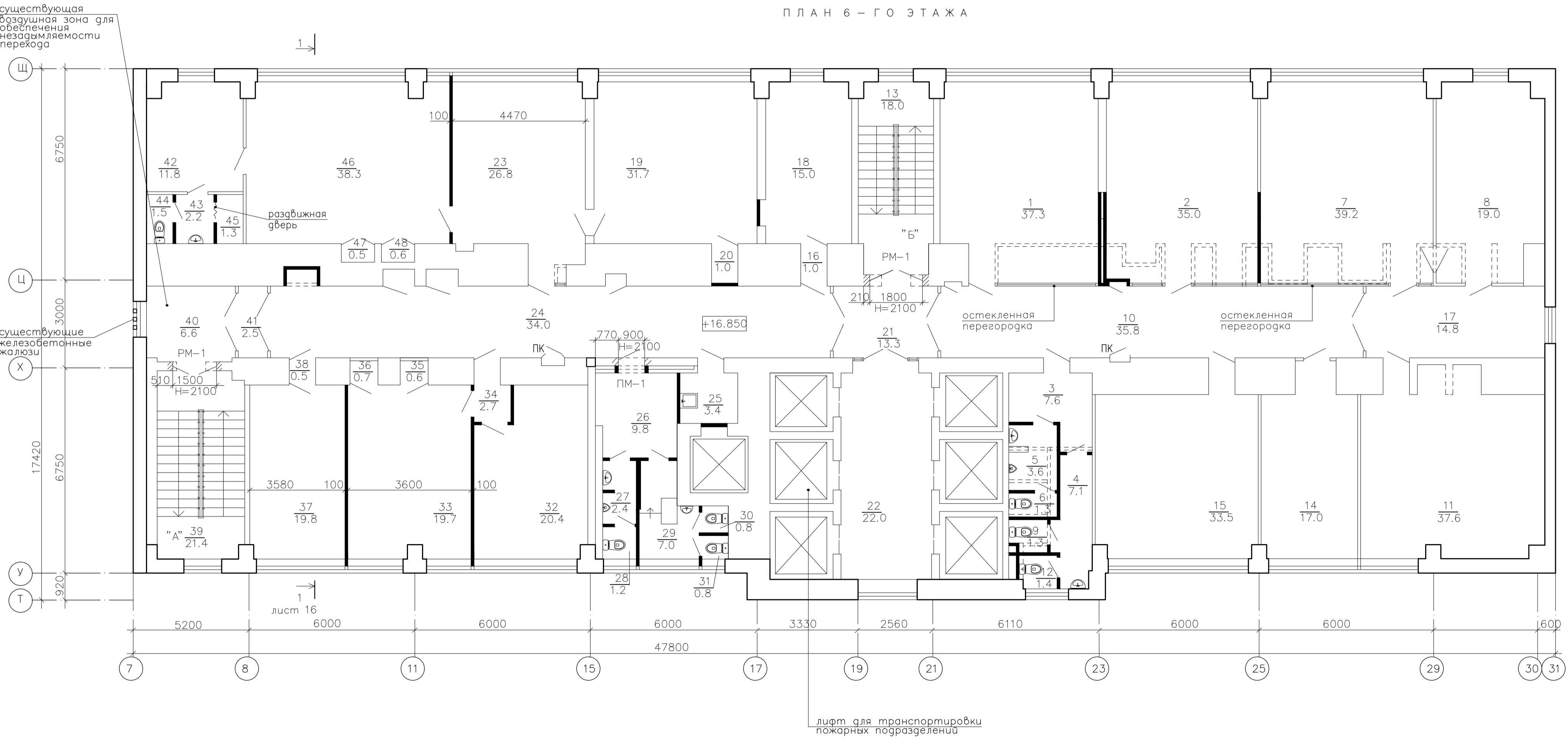
ПЛАН 6 - ГО ЭТАЖА
