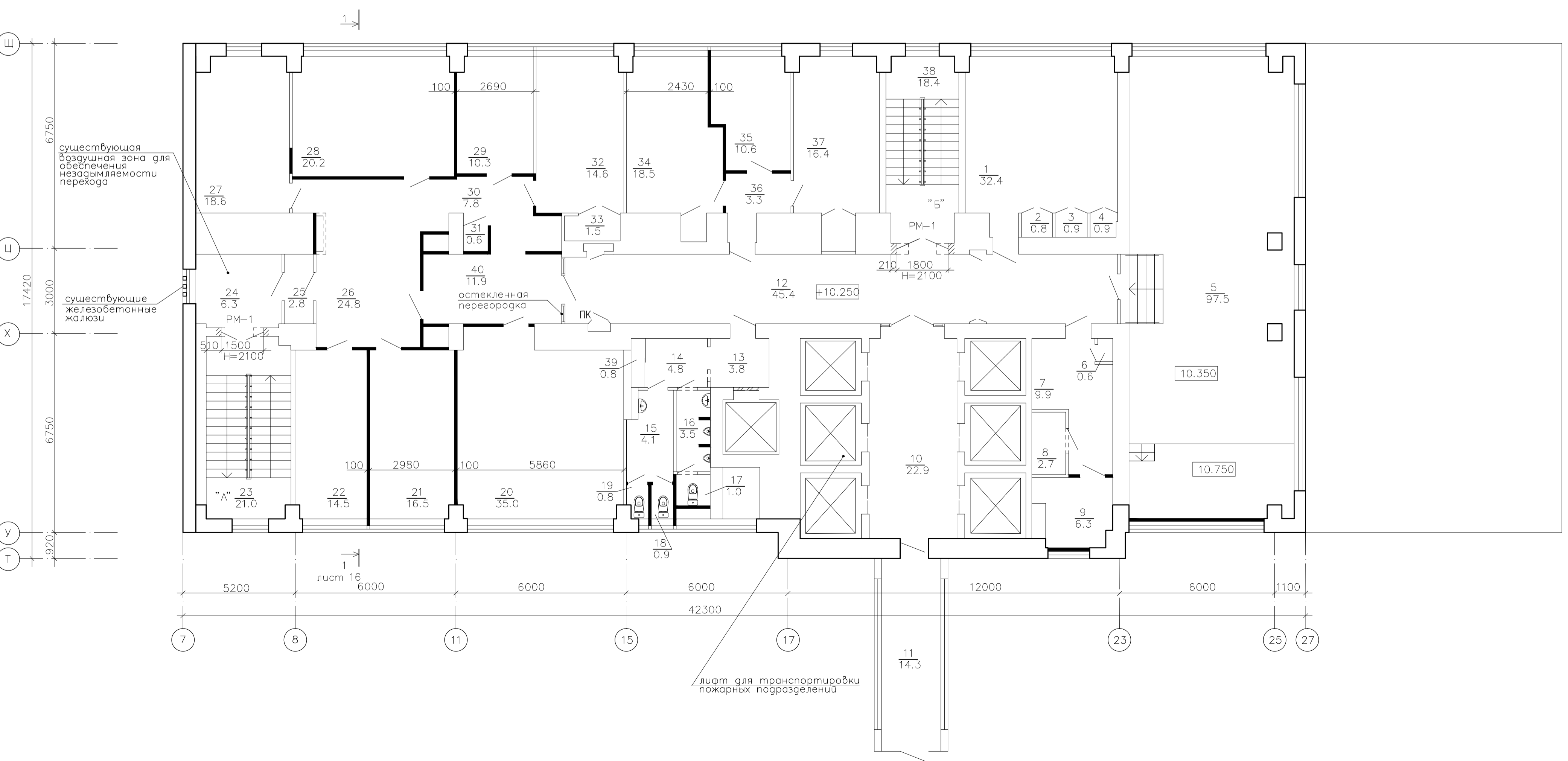
ПЛАН 4 – ГО ЭТАЖА
