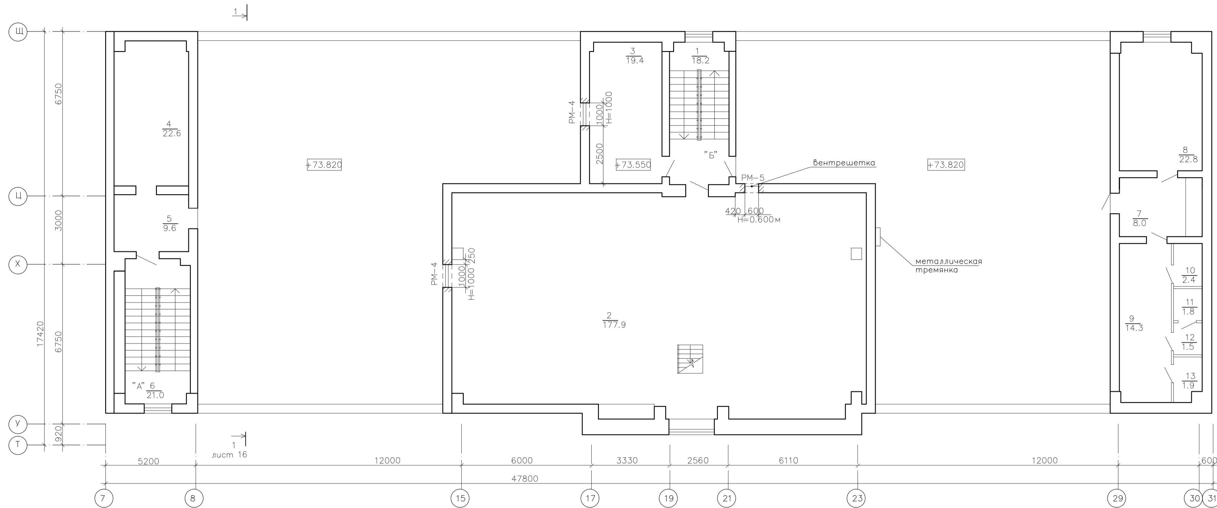
ПЛАН ТЕХНИЧЕСКОГО ЭТАЖА НА ОТМ.+73.550М
