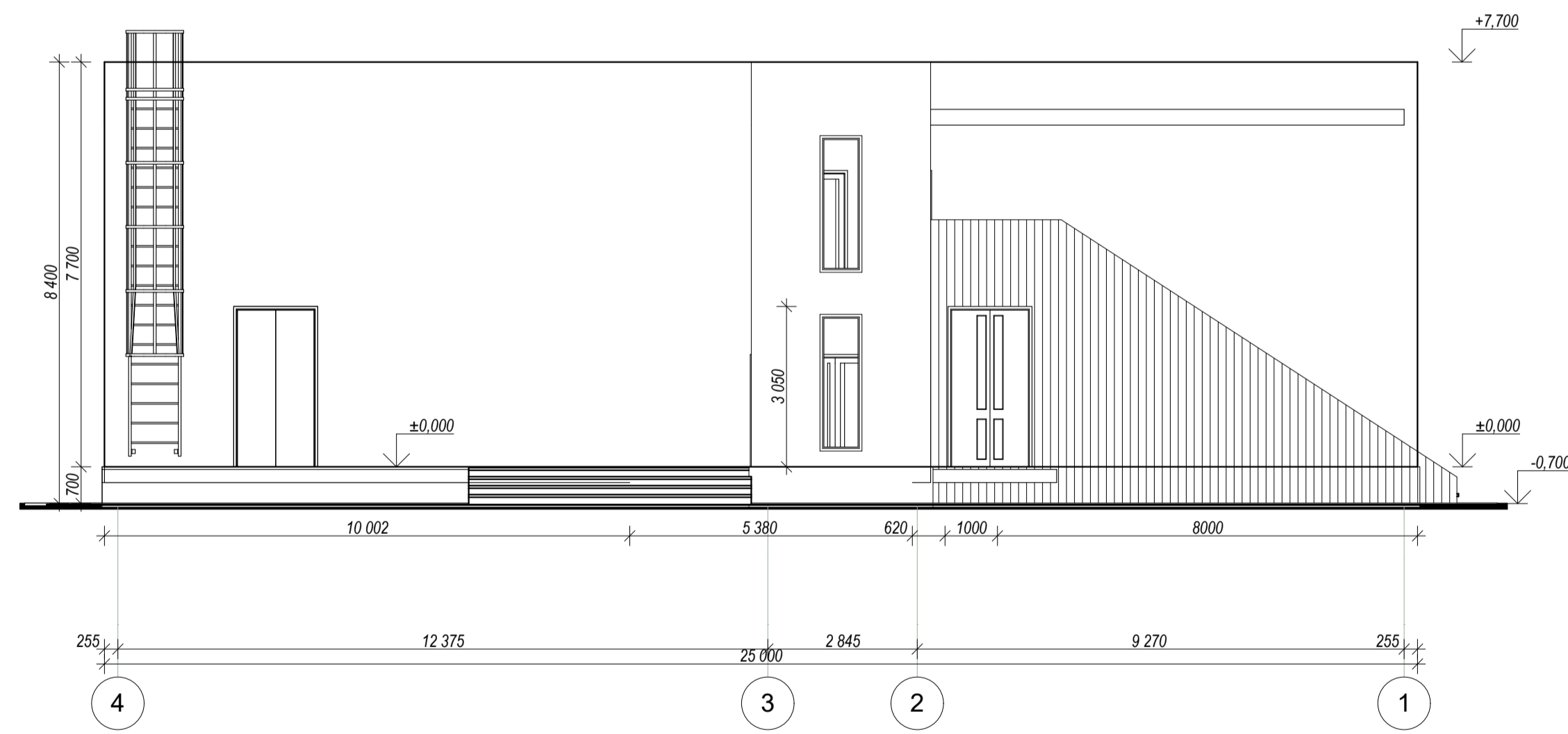
Фасад в осях 4-1.
