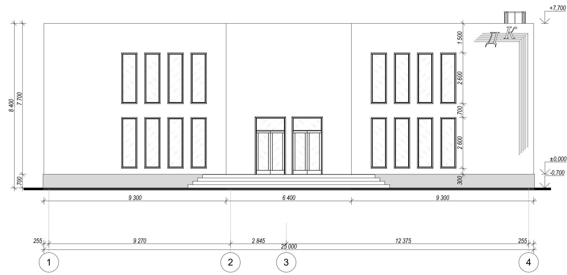
Фасад в осях 1-4.
