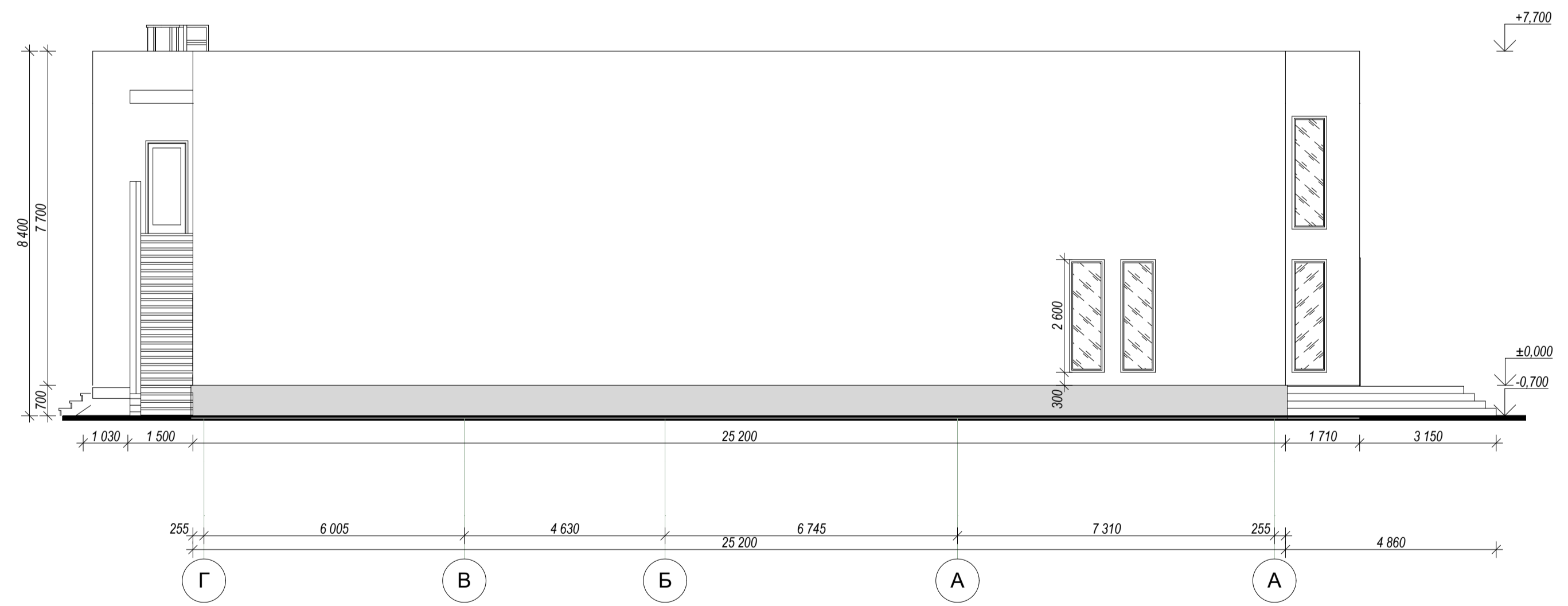
Фасад в осях Г-А.
