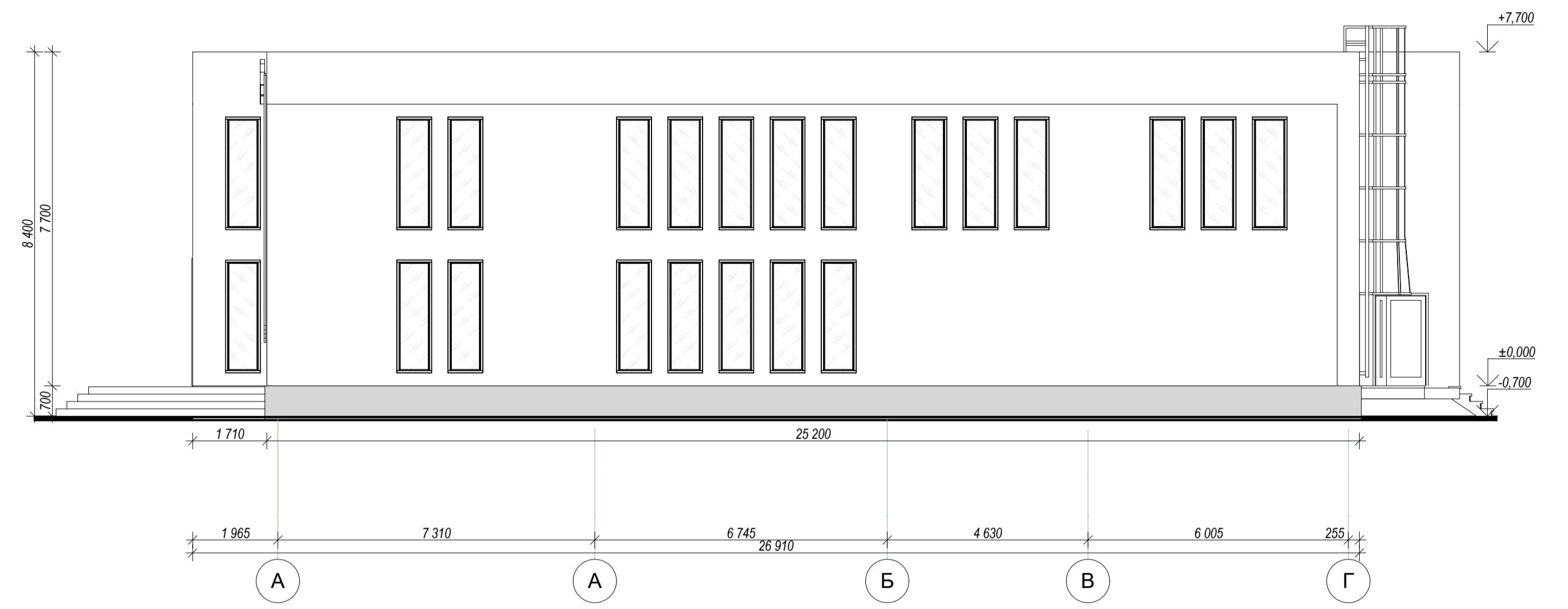
Фасад в осях А-Г.
