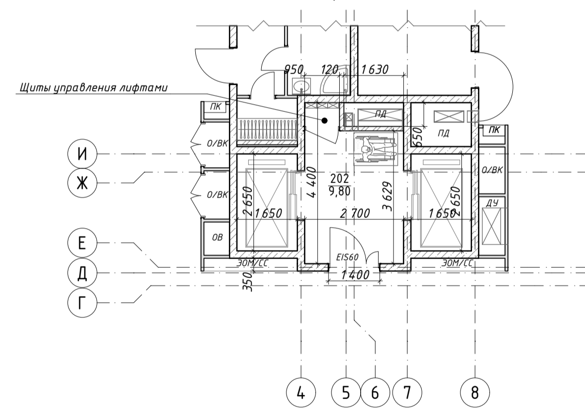
Фрагмент плана 13 этажа. Размещение щитов управления лифтами
