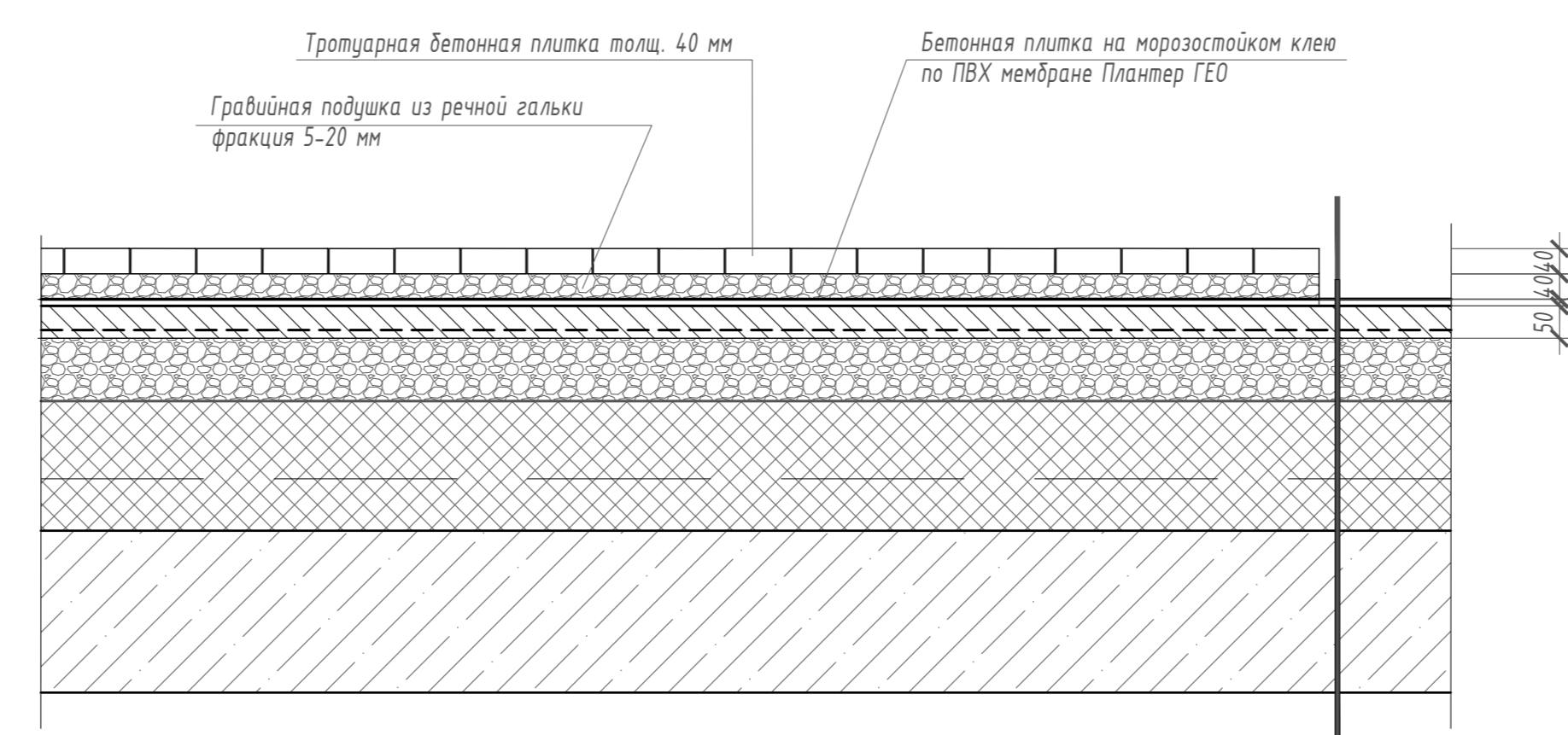
Узел устройства тротуарной плитки на кровле м 1:10
