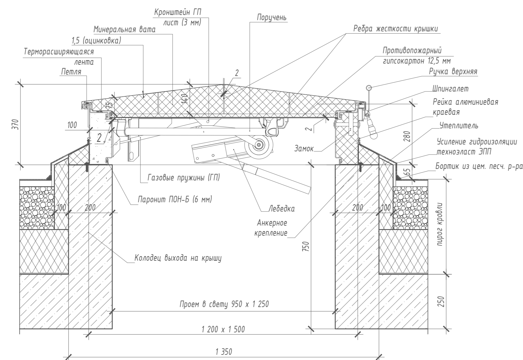
Узел устройства лека выхода на кровлю м 1:10
