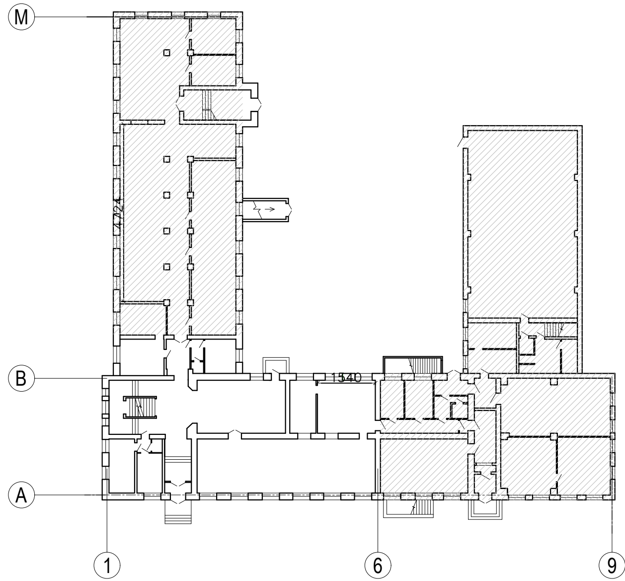
Компоновочный план 1-го этажа
