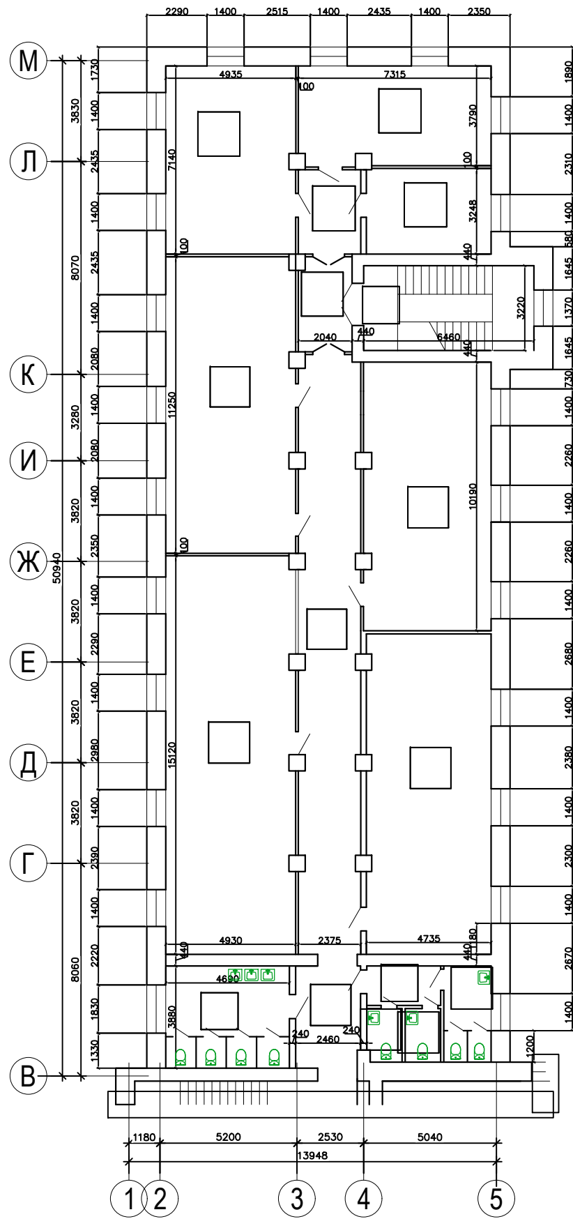
Фрагмент плана 2-го этажа в осях В-М/1-5 (проект)
