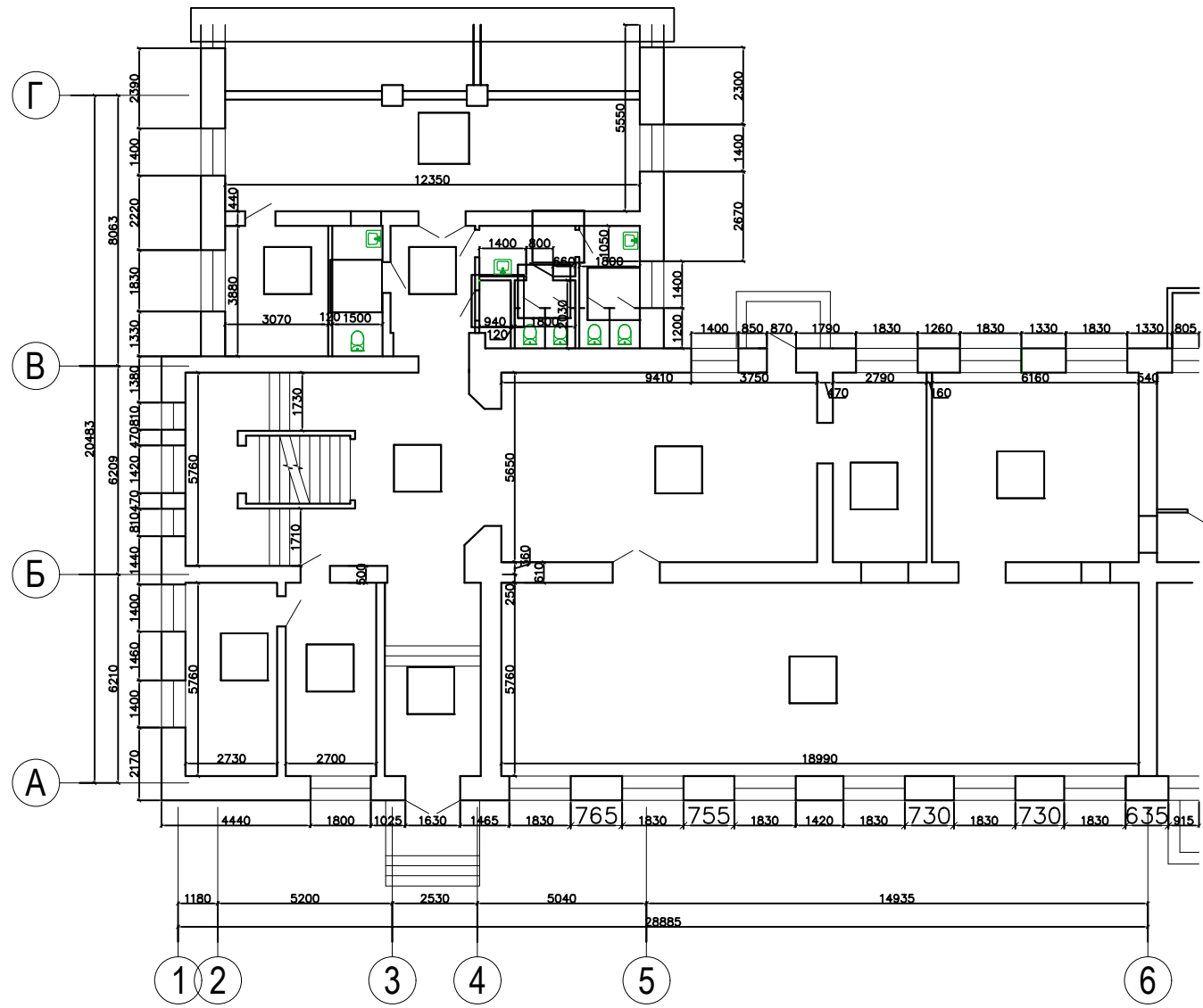
Фрагмент плана 1-го этажа в осях А-Г/1-6 (проект)
