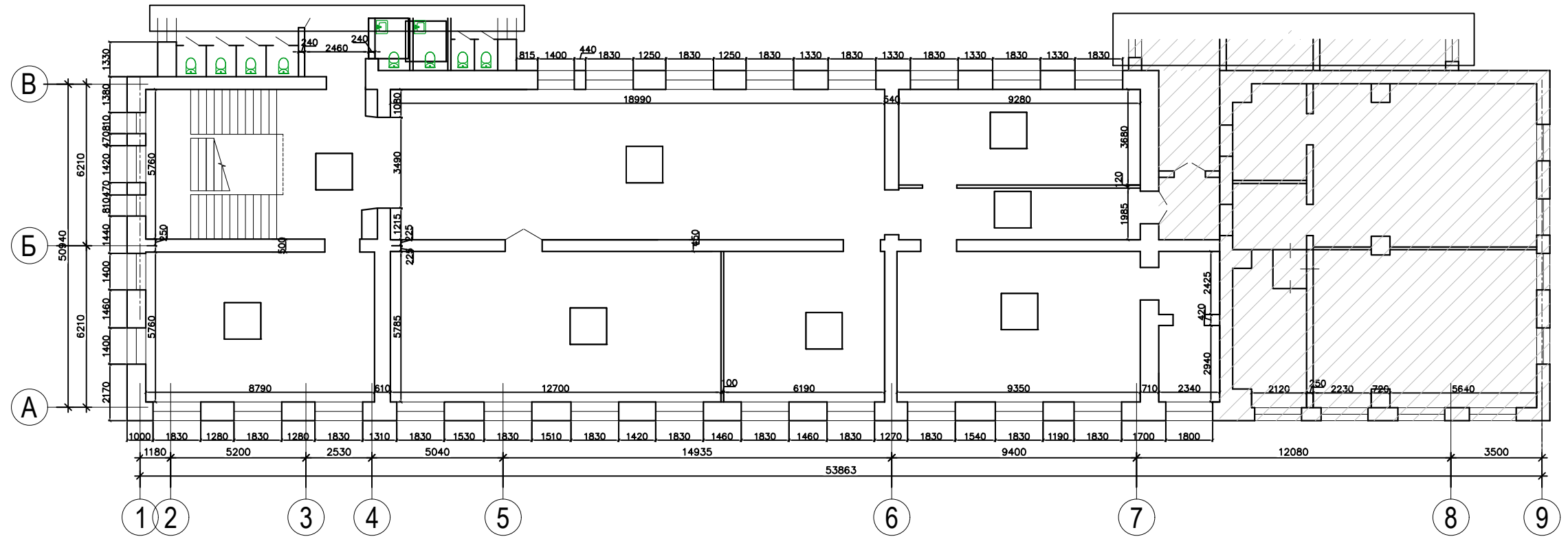
Фрагмент плана 2-го этажа в осях А-В/1-9 (проект)
