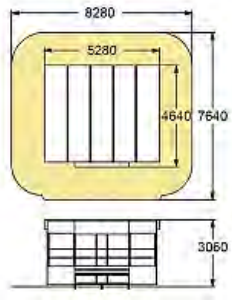
Теневой навес 5x4
