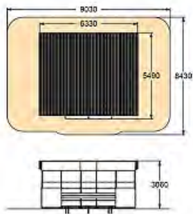
Теневой навес 6x5
