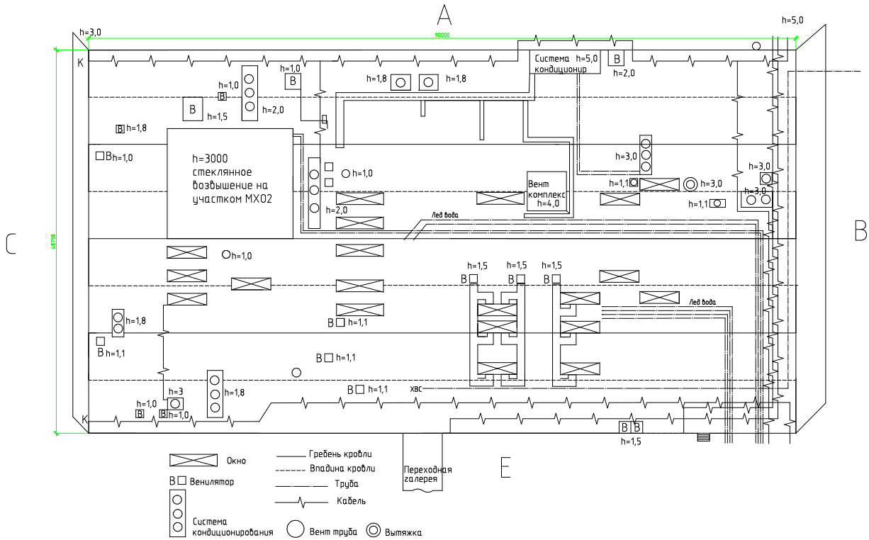
Схема предполагаемой скатной кровли в развертке
