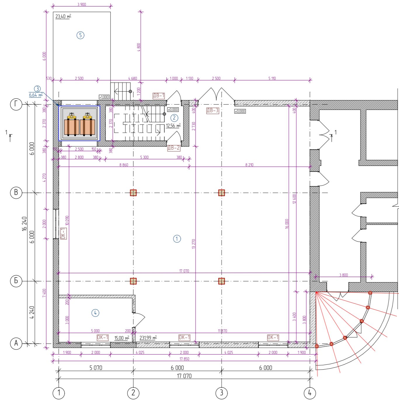
План 1 этажа, М 1:150
