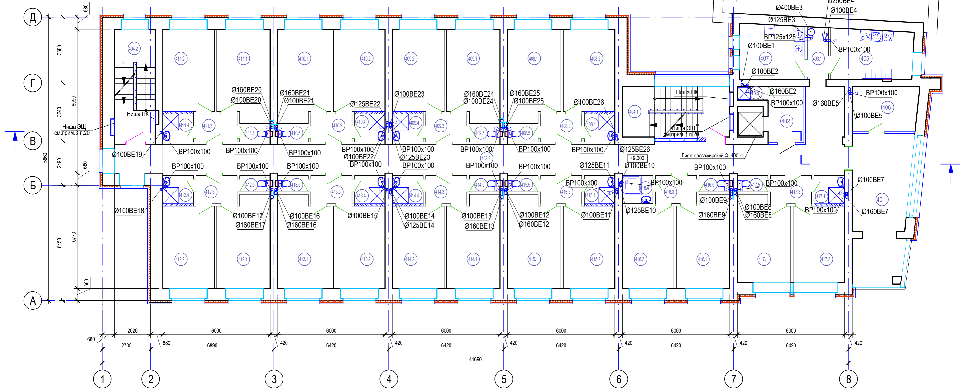
Экспликация помещений 4 этажа (начало)
