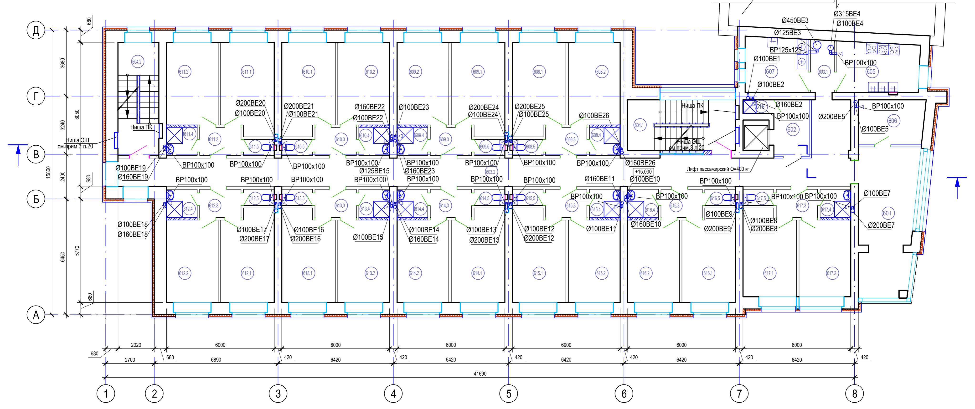
Экспликация помещений 6 этажа (начало)
