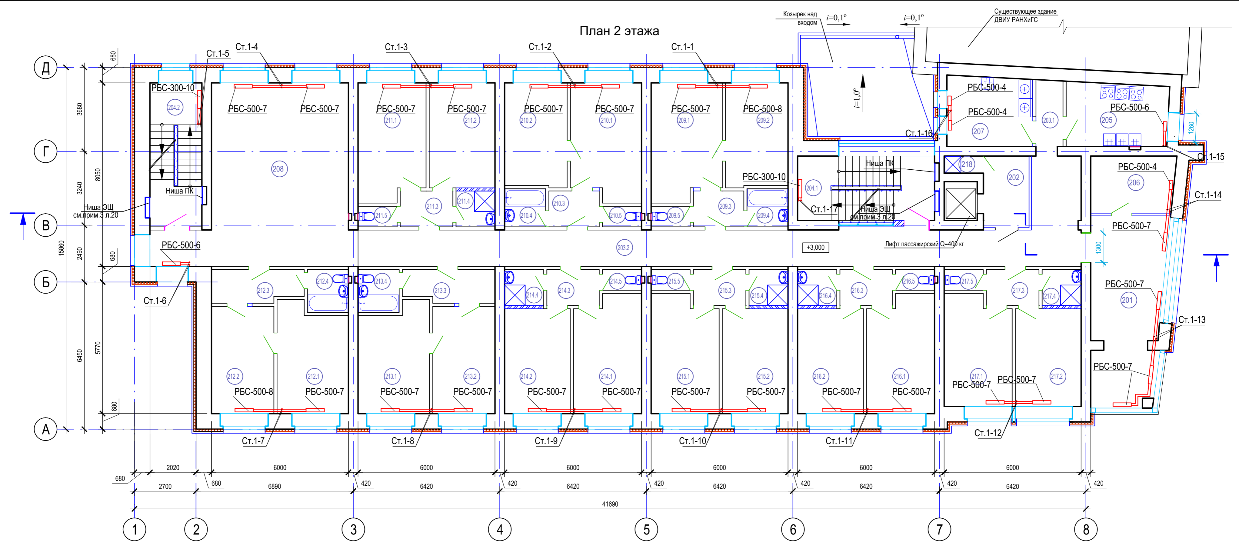
Экспликация помещений 2 этажа (начало)
