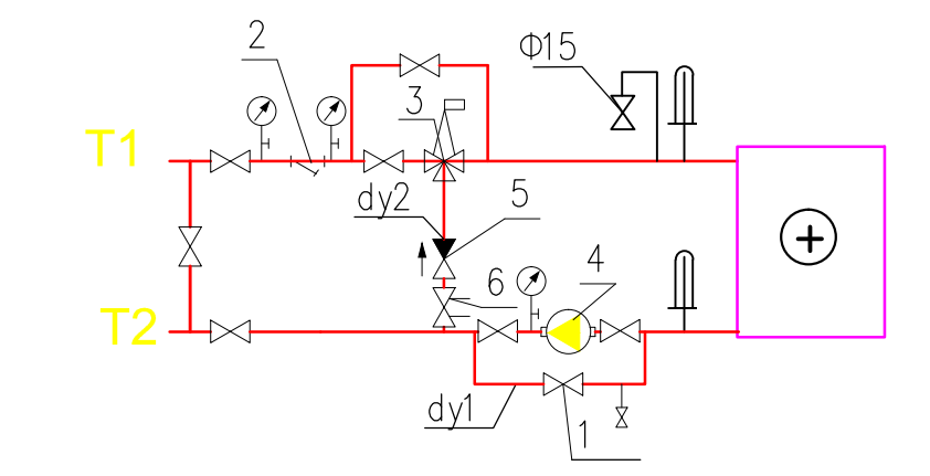
Принципиальная схема обвязки calorifiers (in case of installation without a complete connection)
