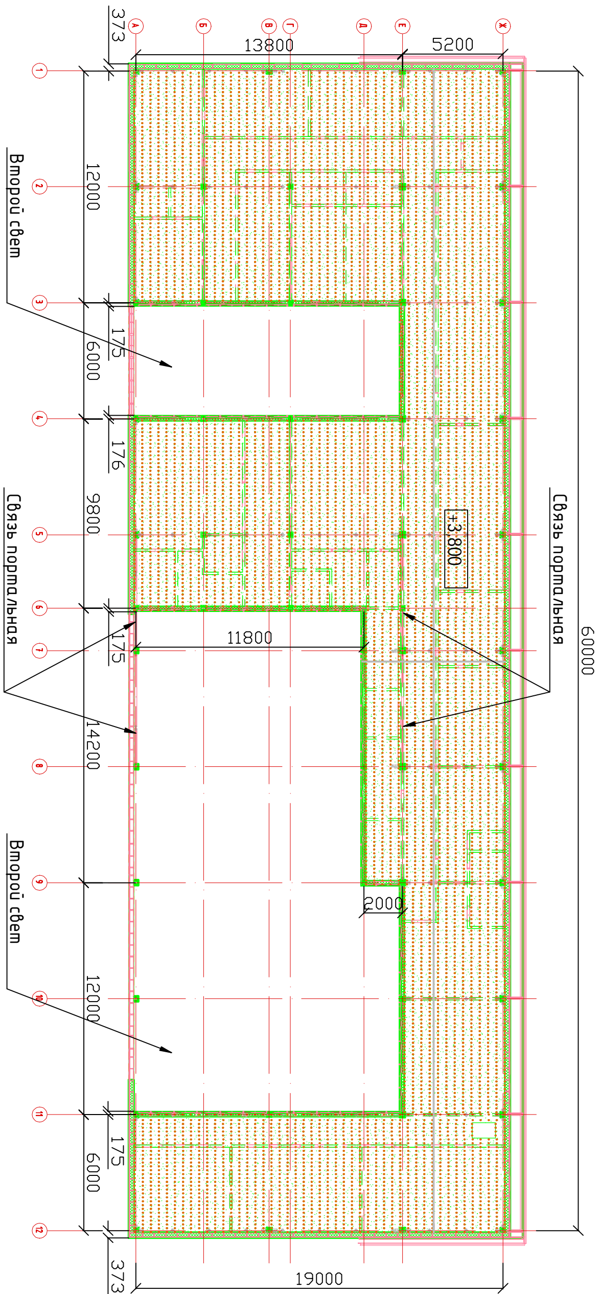
План перекрытия на отм. +3.800 м
