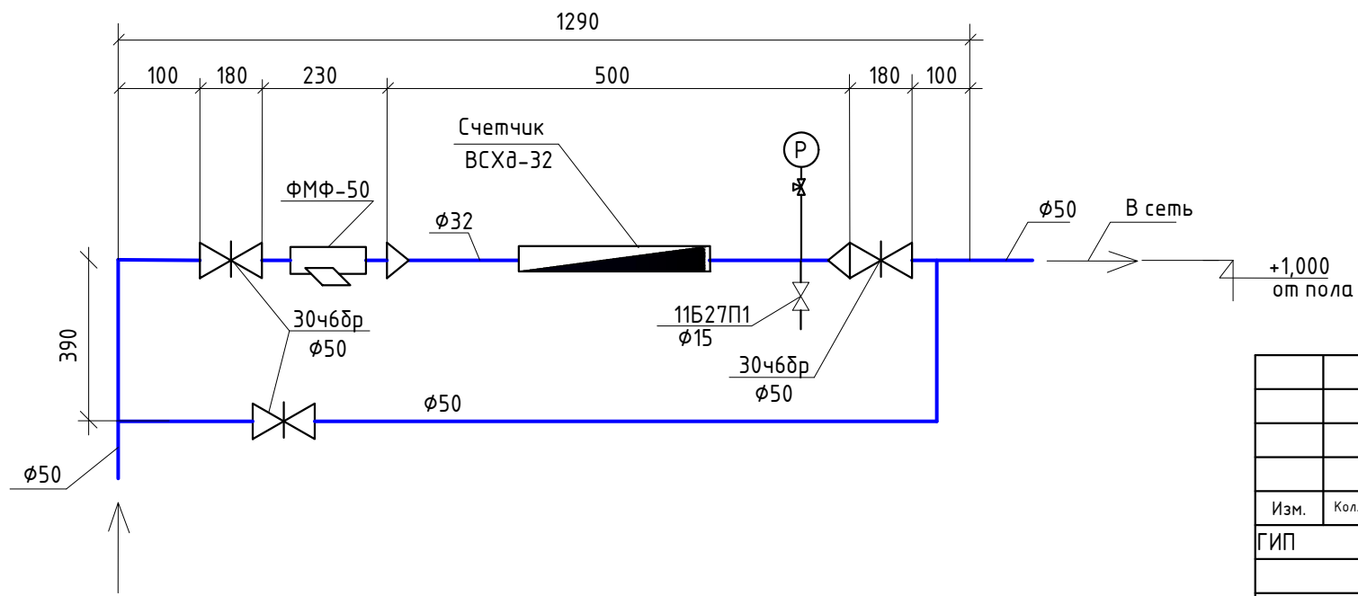
Схема водомерного узла В1
