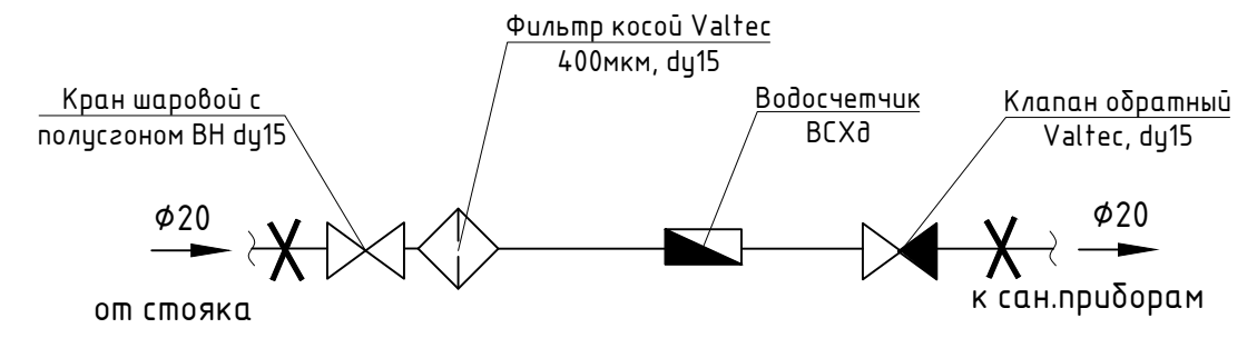
Схема поквартирного водомерного узла
