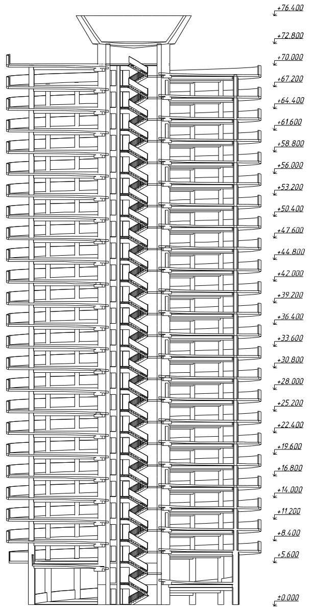
Разрез 1-1
