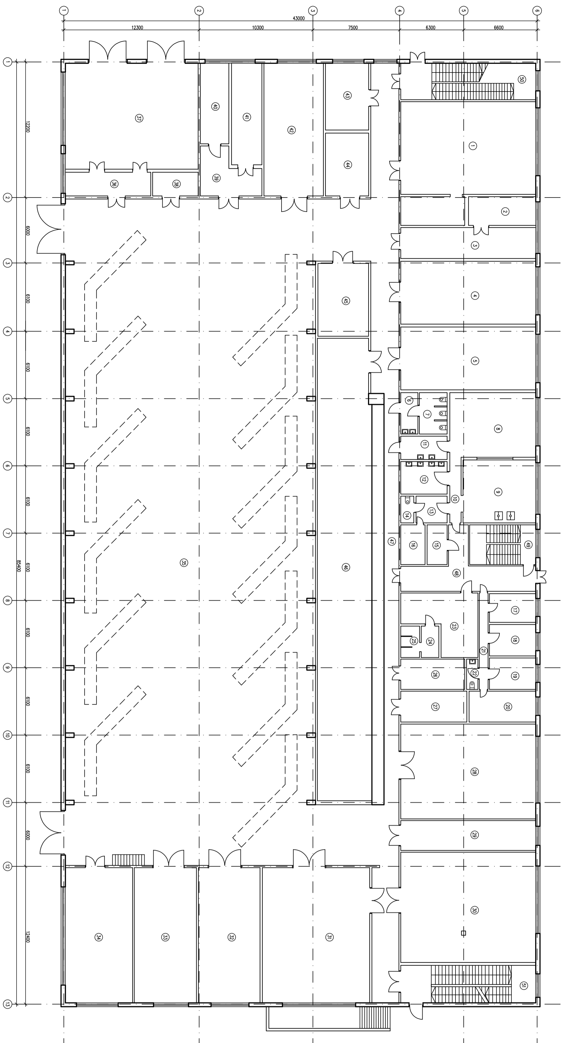
План 1-го этажа М 1:100
