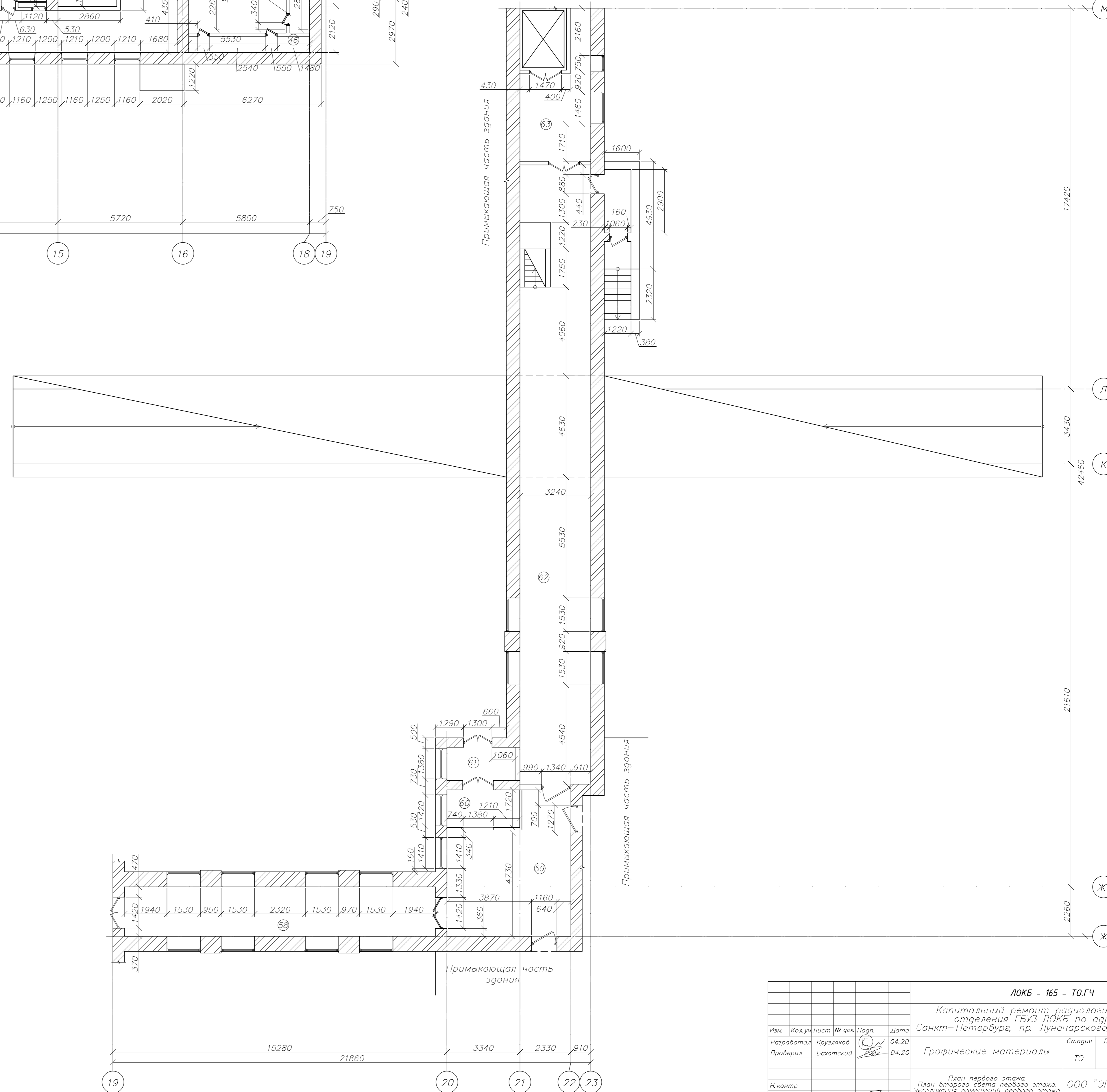
План первого этажа (участок в осях 19-23)
