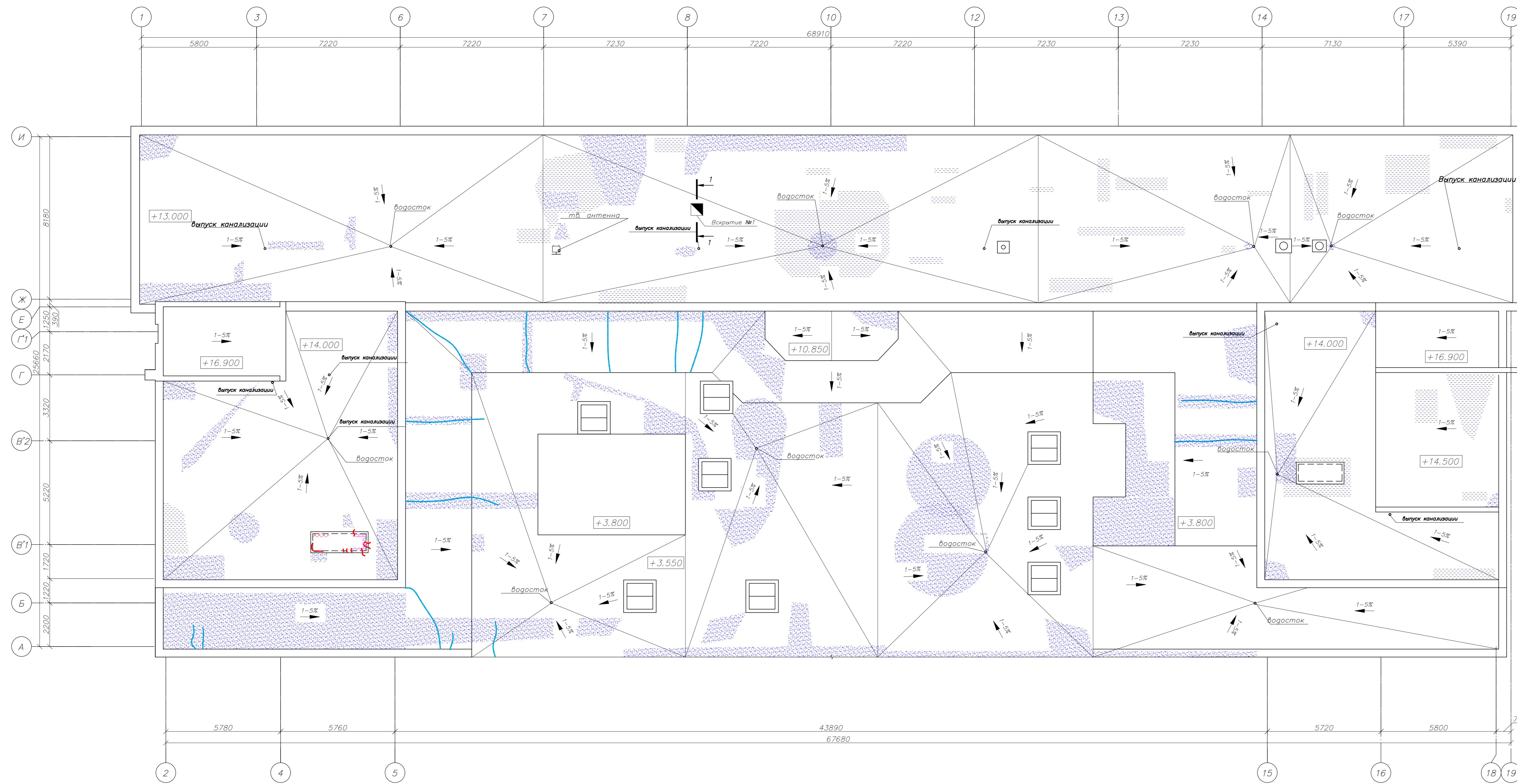
План кровли с обозначением дефектов (участок в осях 1-19)
