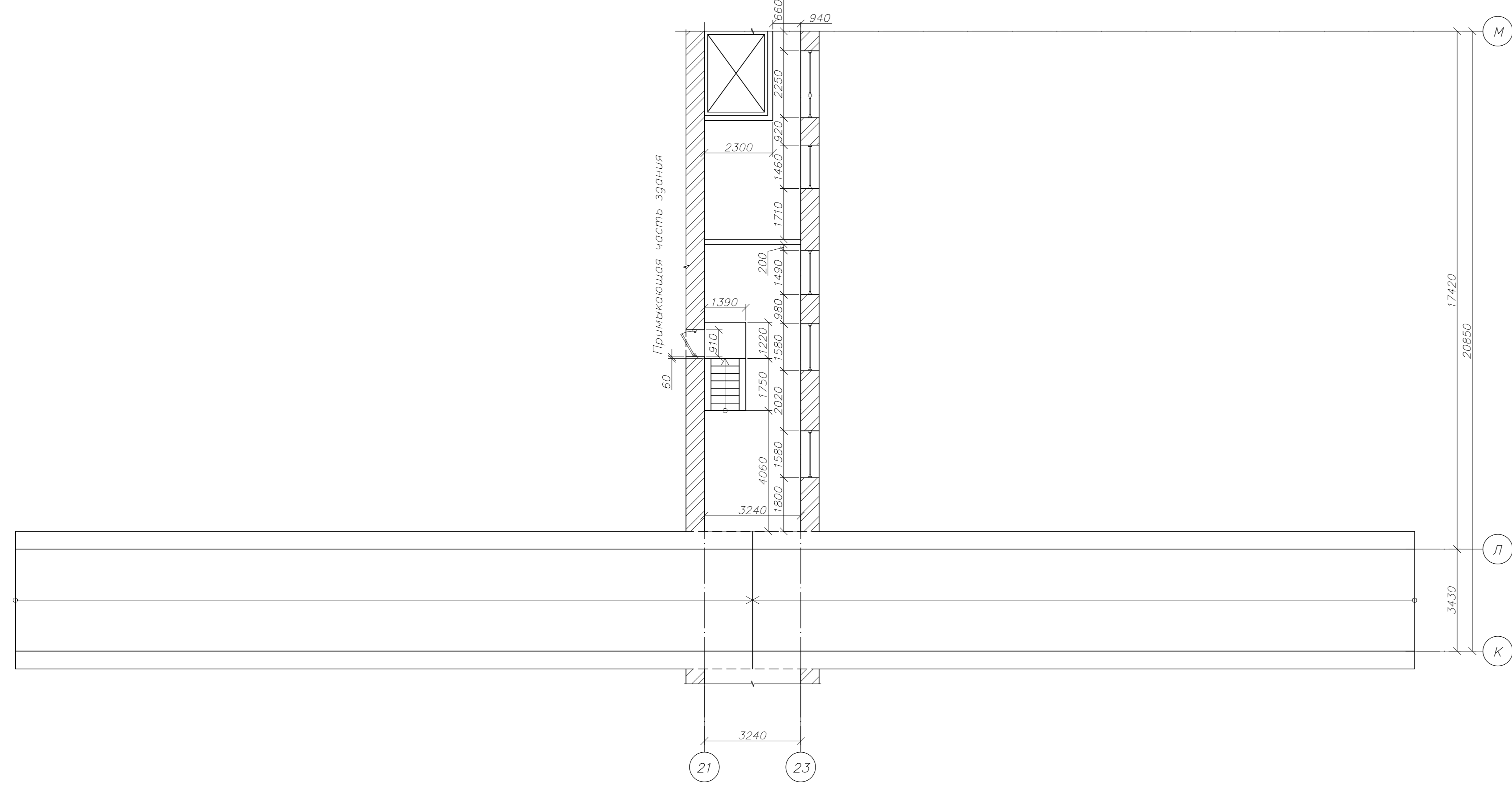
Экспликация помещений первого этажа (участок в осях 19-23)
