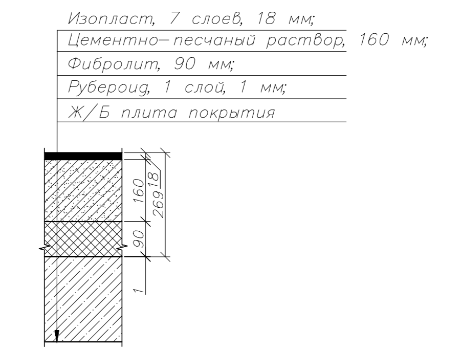
Вскрытие №1. Разрез 1-1
