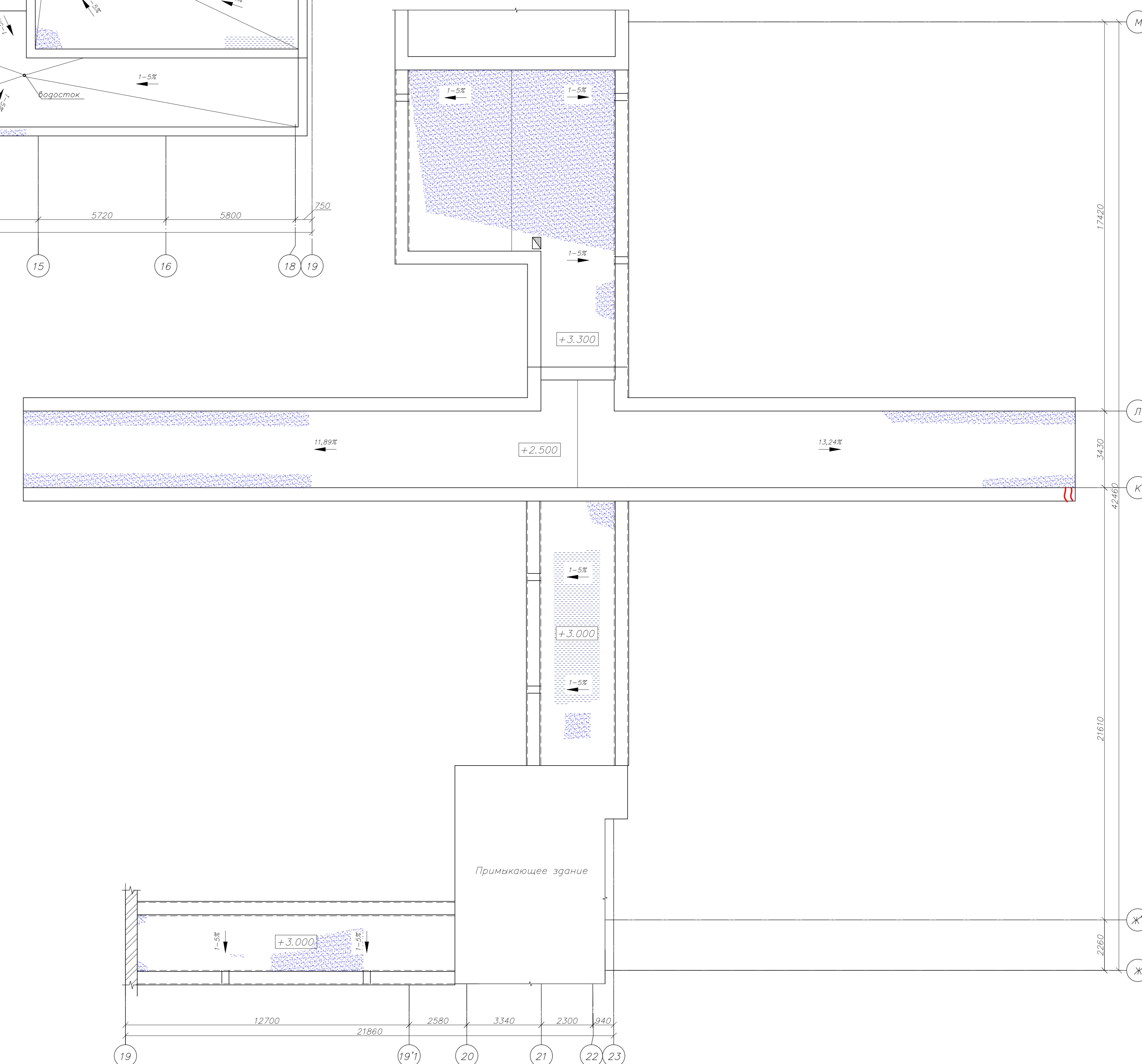
План кровли с обозначением дефектов (участок в осях 19-23)
