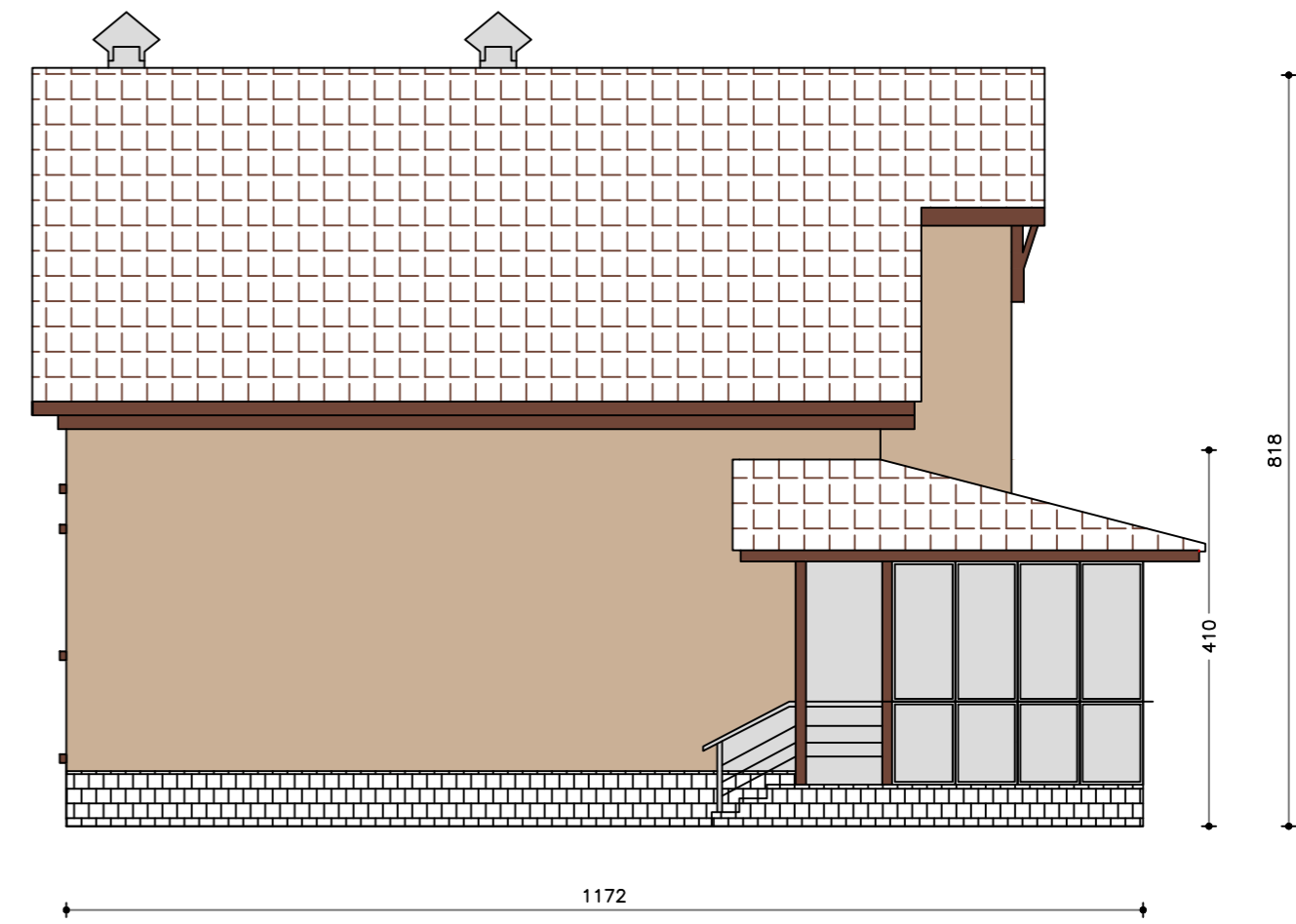
Вид слева
