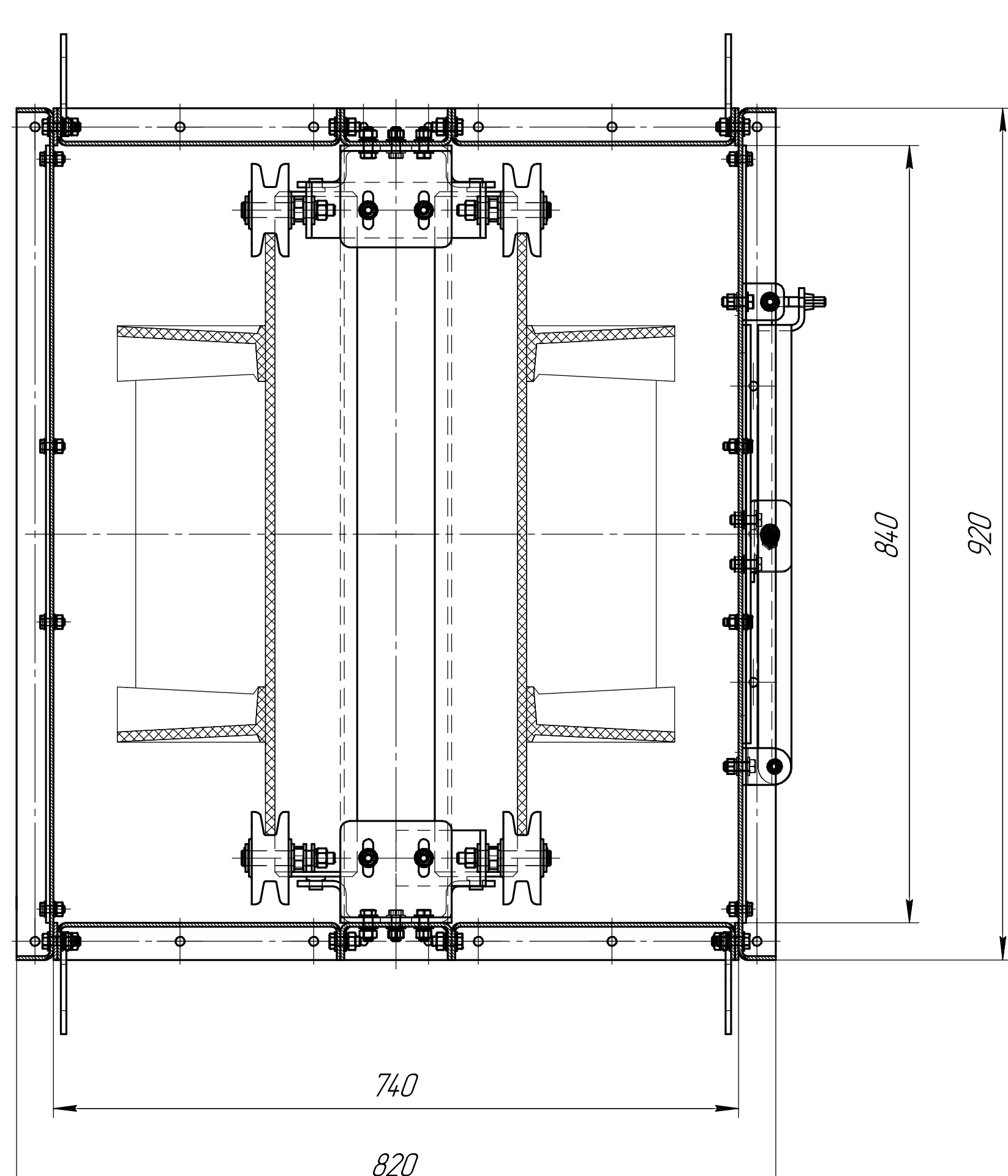
И-И(1:5)
