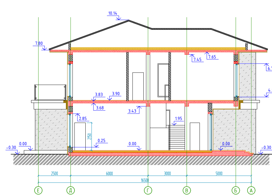
РАЗРЕЗ 2-2
