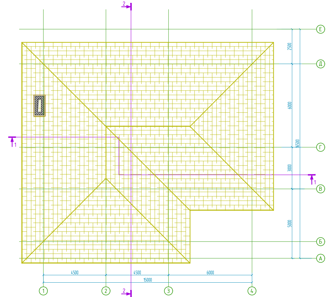
ПЛАН КРОВЛИ
