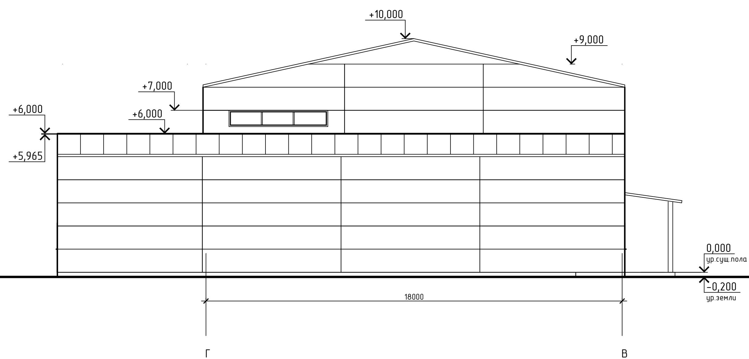
ФАСАД Г - В
