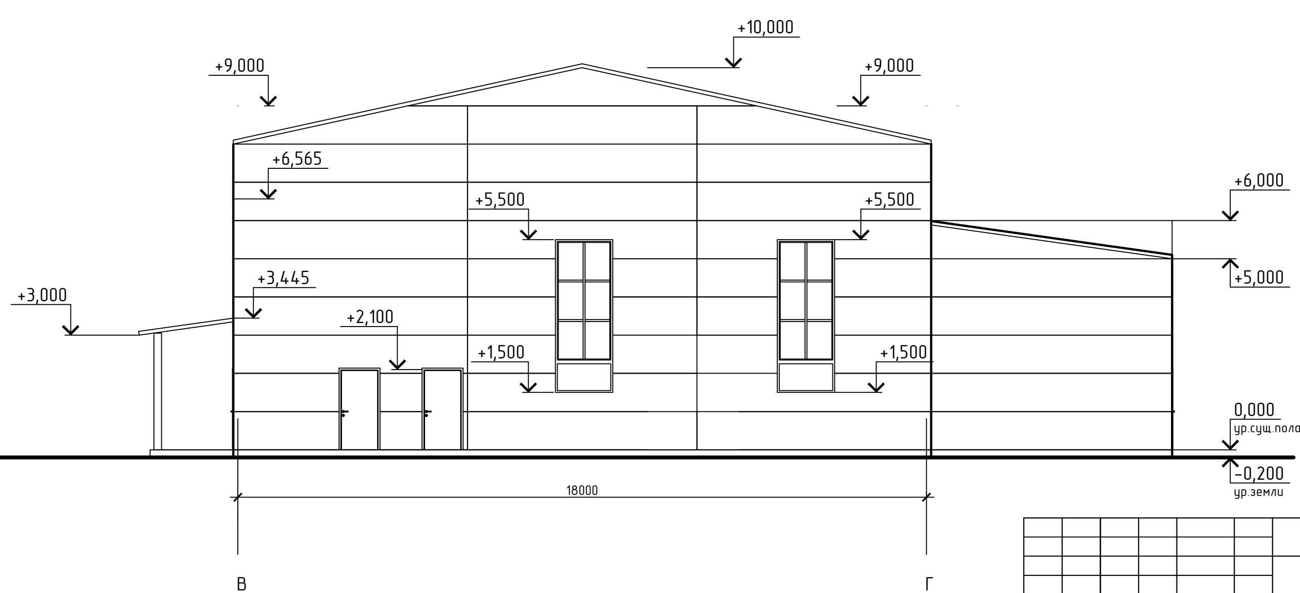
ФАСАД В - Г
