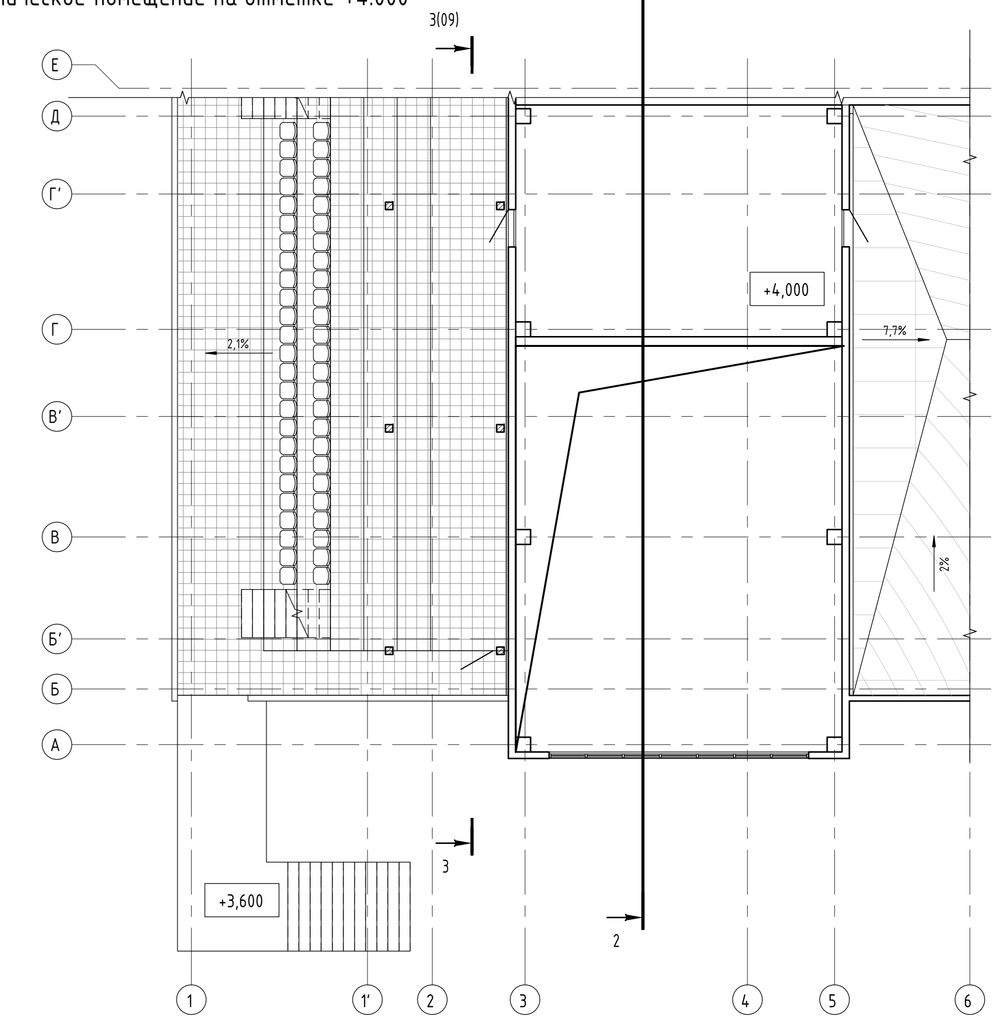
Техническое помещение на отметке +4.000
