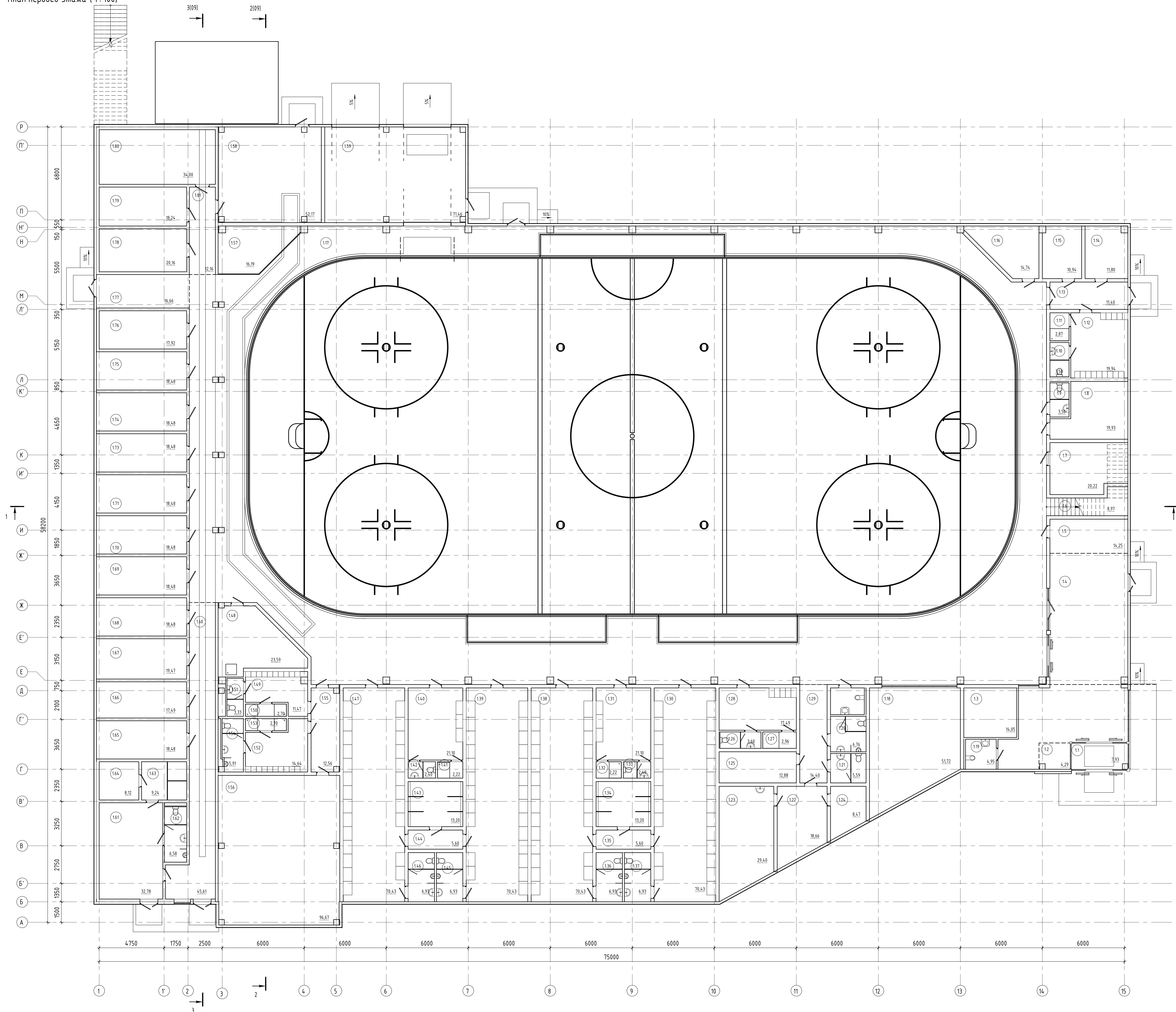
План первого этажа (1:100)
