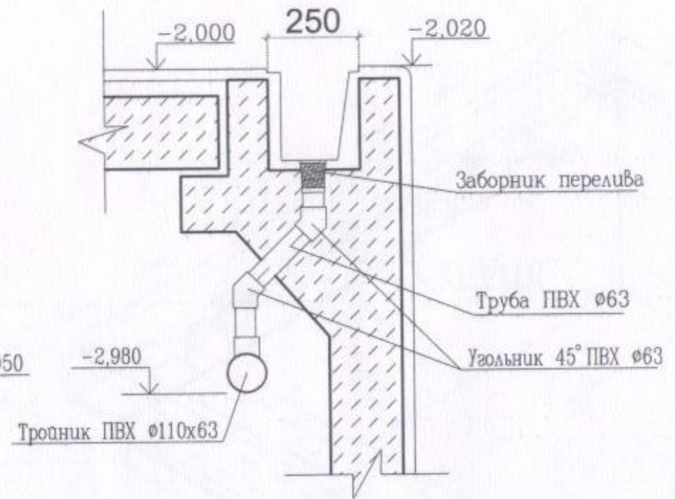
Разрез 2 - 2 заборник воды
