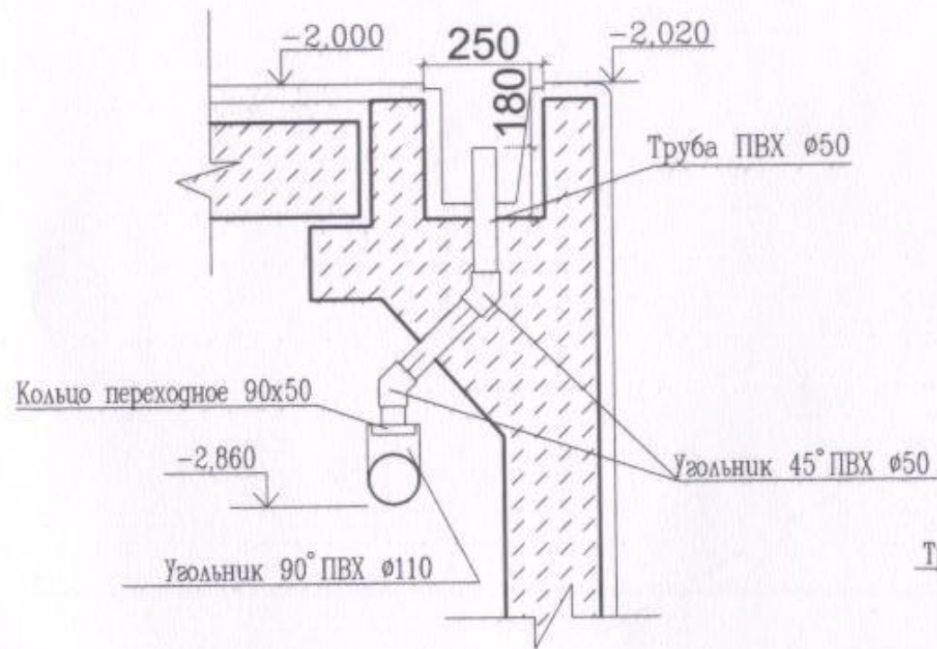
Разрез 1 - 1 заборник воздуха
