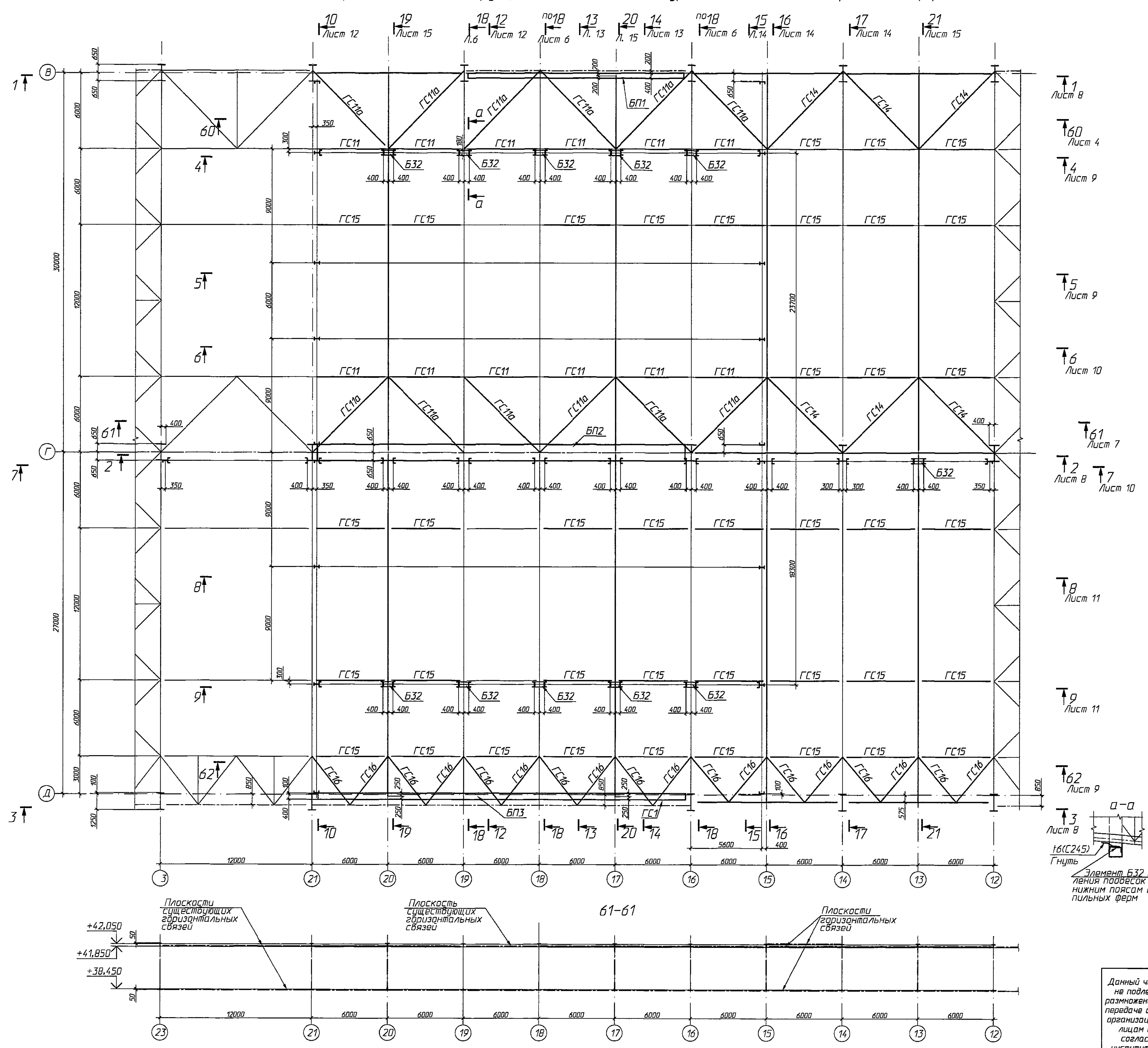
Схема расположения конструкций вытяжного зонта в уровне нижних поясов стропильных ферм
