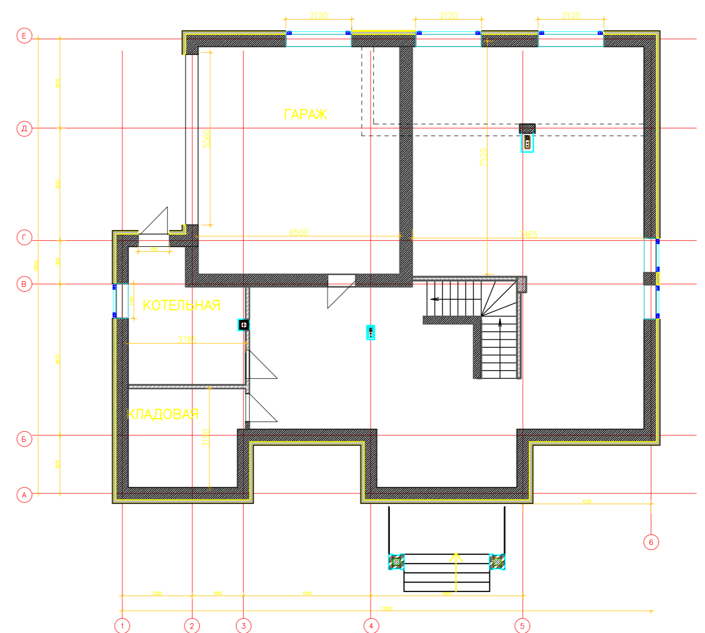
ЦОКОЛЬ
