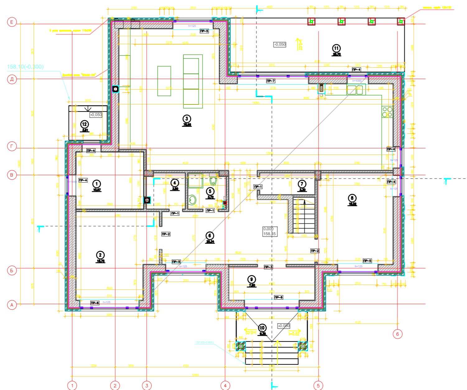
1 ЭТАЖ
