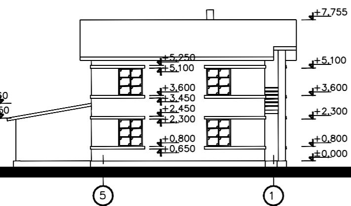
Фасад 5-1 (М 1:150)
