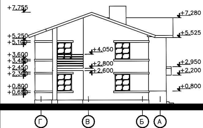
Фасад Г-А (М 1:150)
