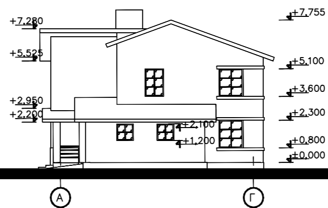
Фасад А-Г (М 1:150)
