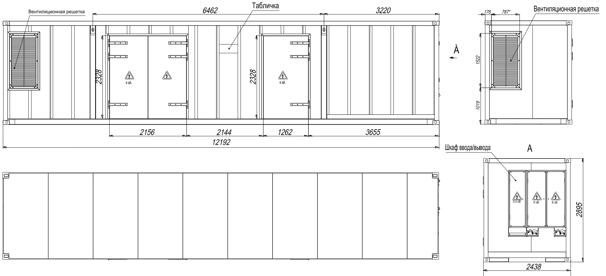
Рисунок Б.1 (лист 1 из 2) – Общий вид, габаритные размеры и компоновка БК
