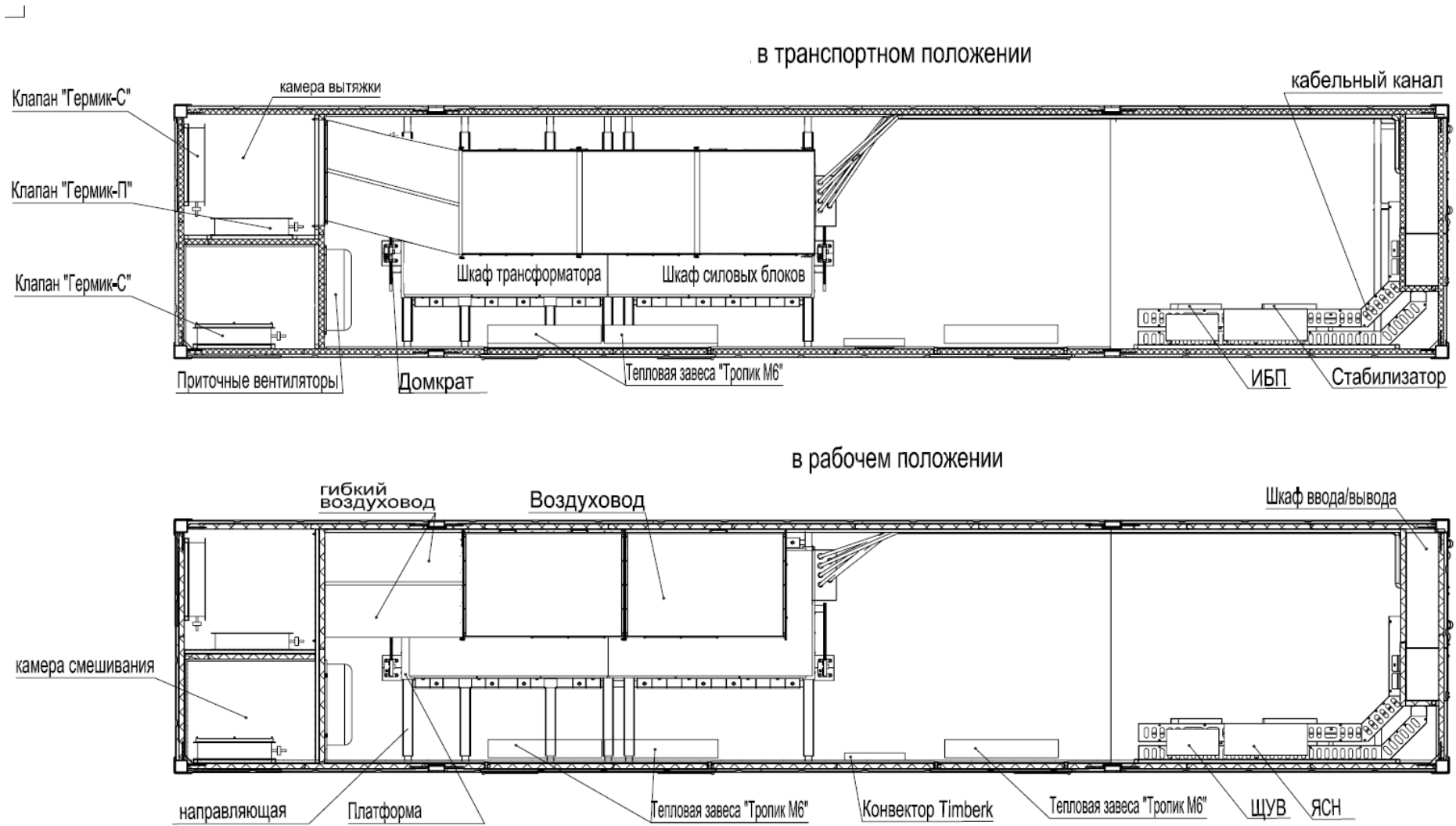
Рисунок Б.1 (лист 2 из 2) – Общий вид, габаритные размеры и компоновка БК
