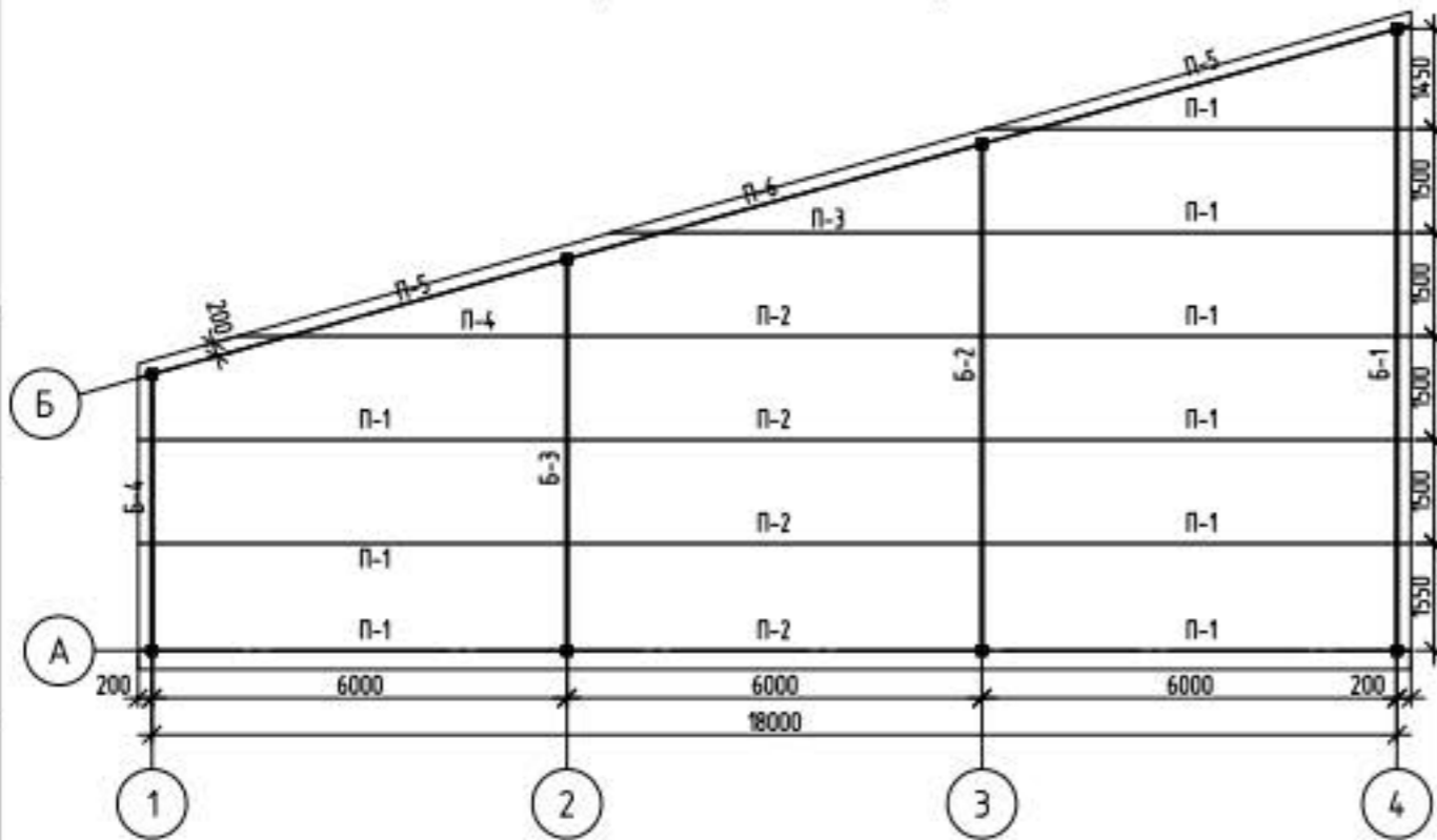
Схема расположения балок и прогонов
