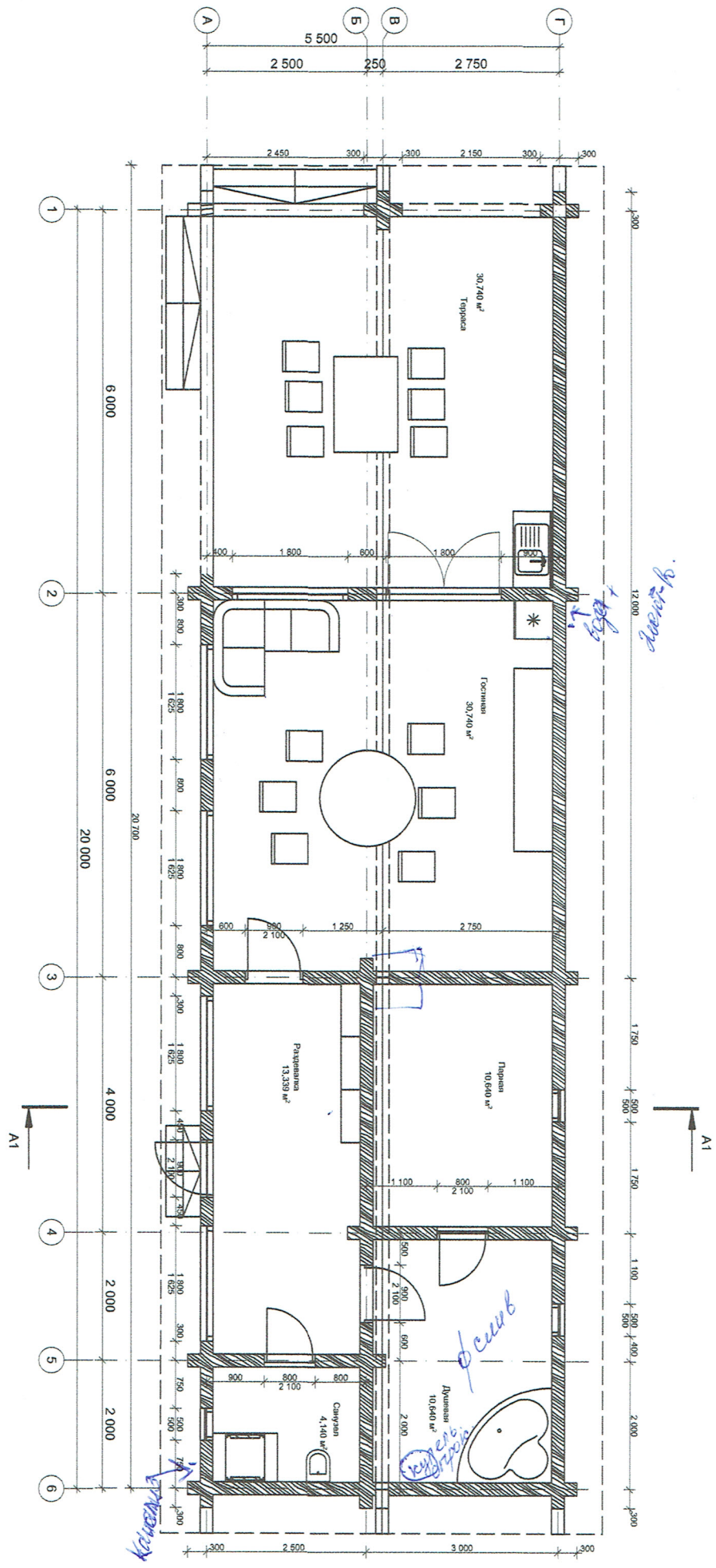
План 1 этажа
