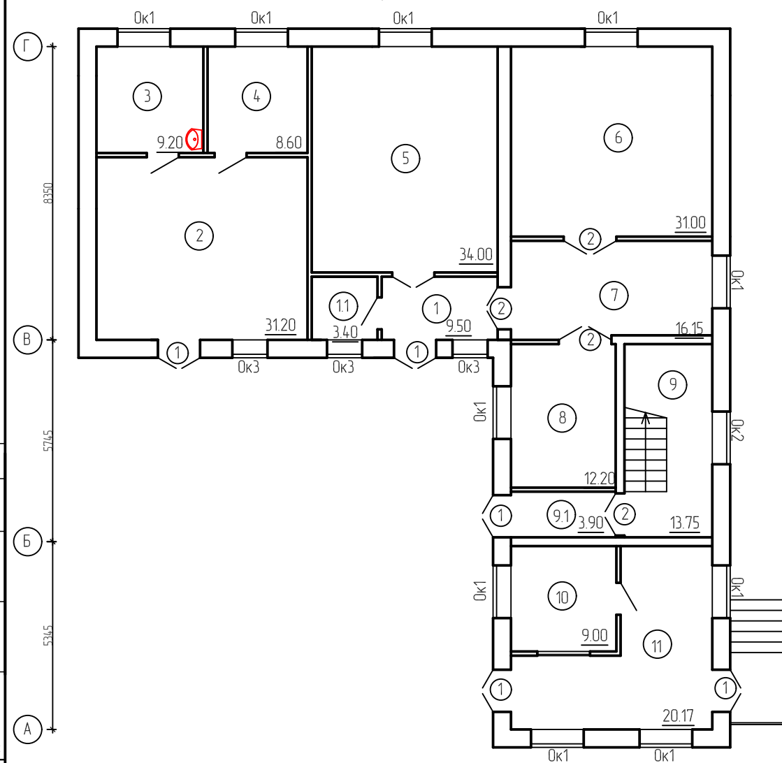
План помещений 1 этажа
