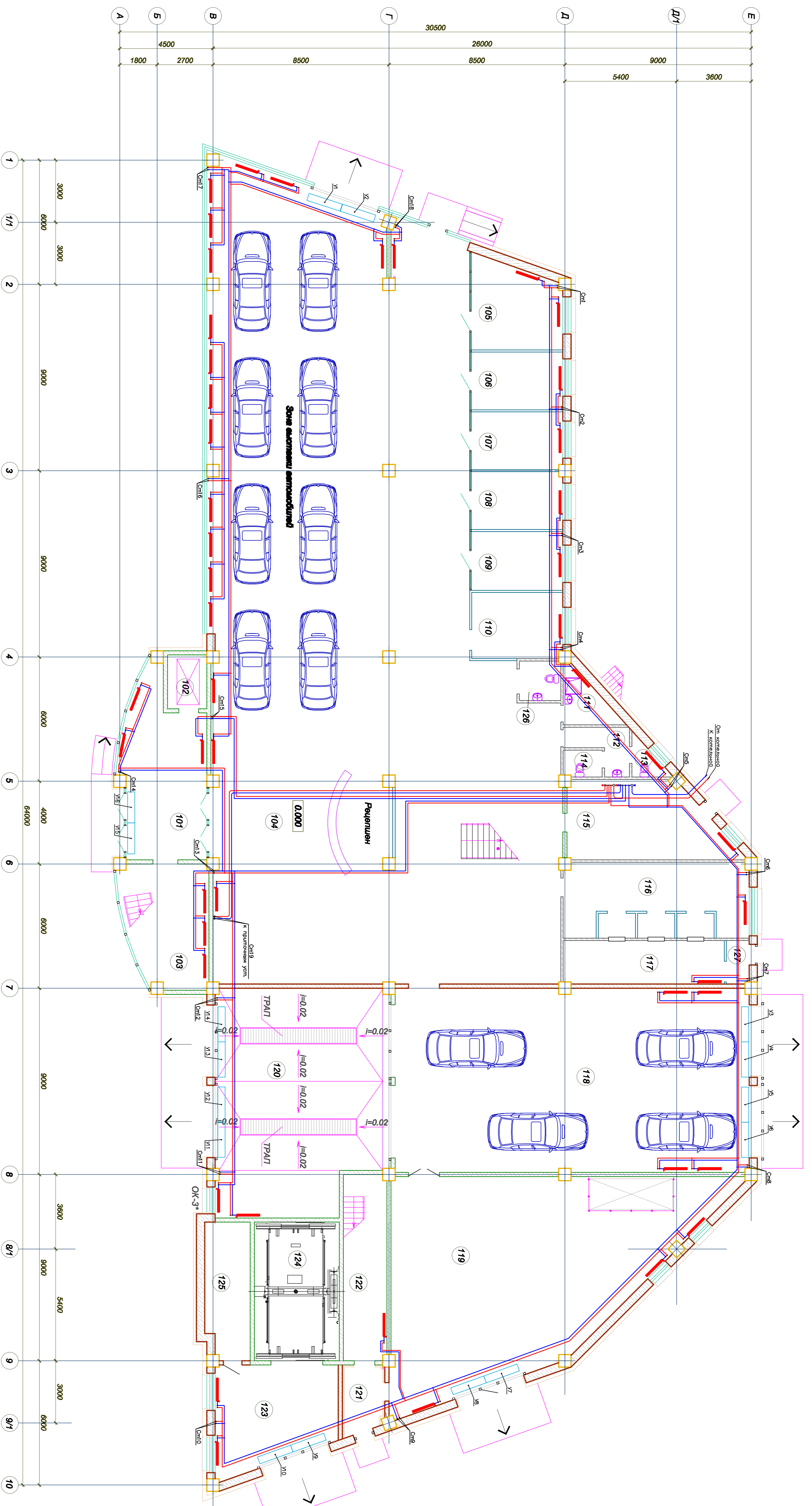
Экспликация помещений на отм. 0.000
