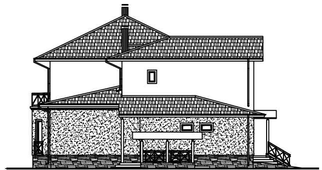
Фасад в осях И-А.
