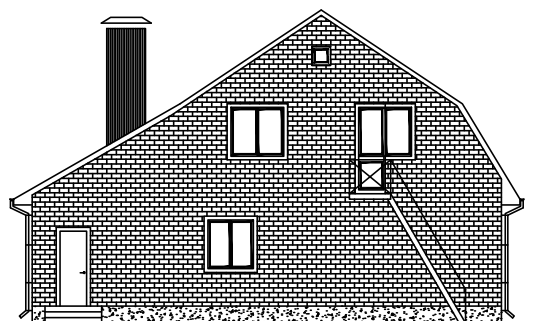
Фасад в осях З-1.
