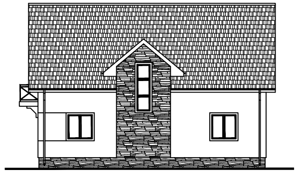
Фасад в осях 5-1.
