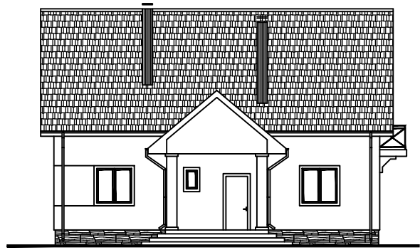
Фасад в осях 1-5.
