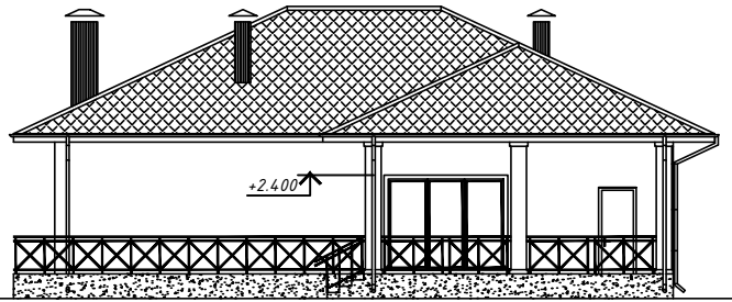
Фасад в осях А-В.
