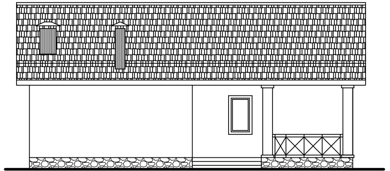
Фасады в осях 1-3.
