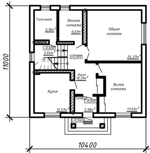
План 1-го этажа.
