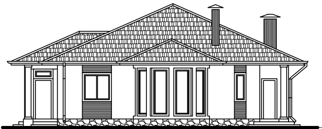
Фасад в осях А-В.
