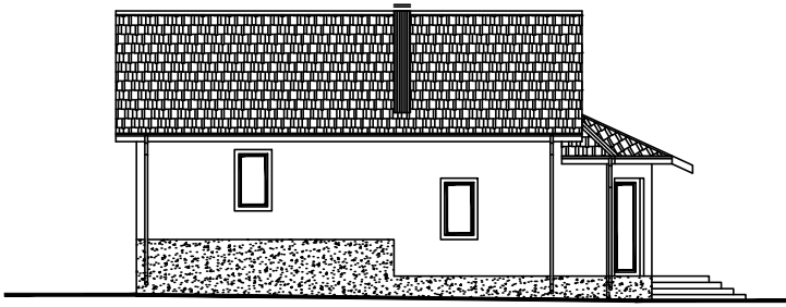
Фасад в осях Д-А.
