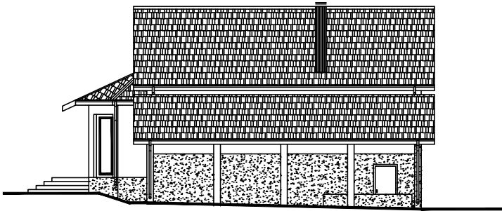
Фасад в осях А-Д.
