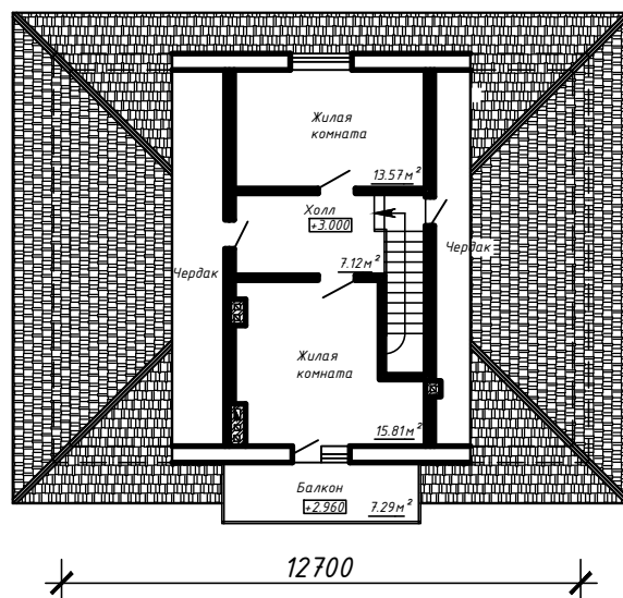
План 2-го этажа.
