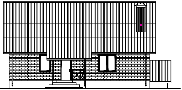
Фасад в осях А-Е.
