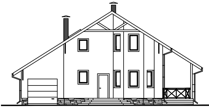
Фасад в осях 1-5.
