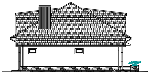
Фасад в осях Г-А.
