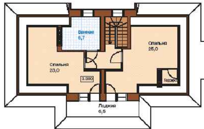
План мансардного этажа
