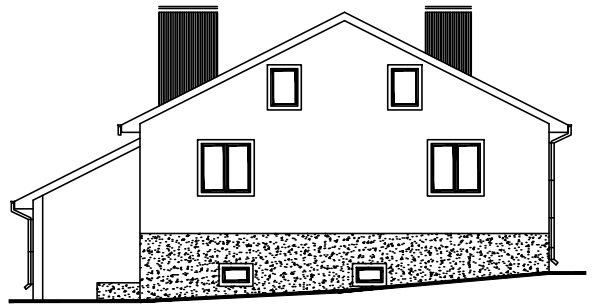
Фасад в осях 5-1.
