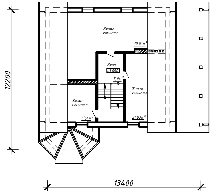
План 2-го этажа.
