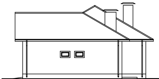
Фасад в осях А-Д.
