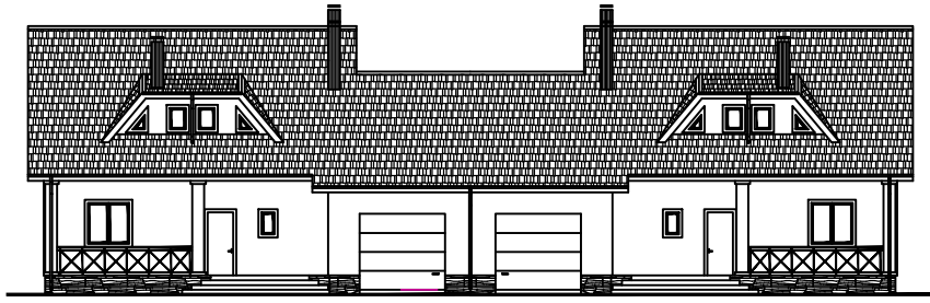
Фасад в осях "1-7".
