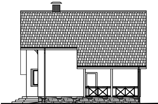
Фасад в осях А-В.
