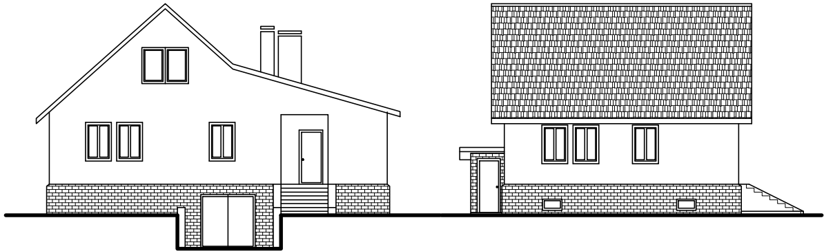
Фасад в осях 1-4.
