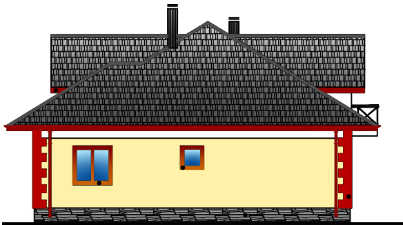
Фасад в осях А-Д.
