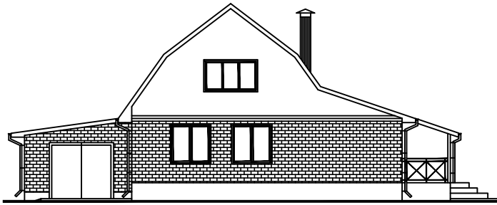
Фасад в осях 1-5.
