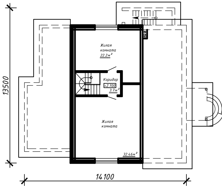
План 2-го этажа.
