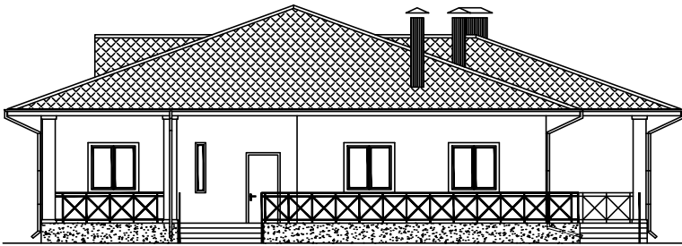
Фасад в осях 1-3.
