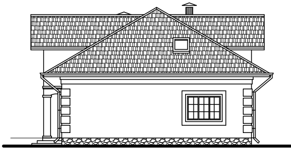
Фасад в осях А-Д.
