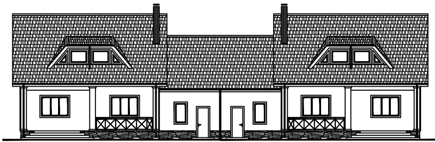
Фасад в осях "7-1".
