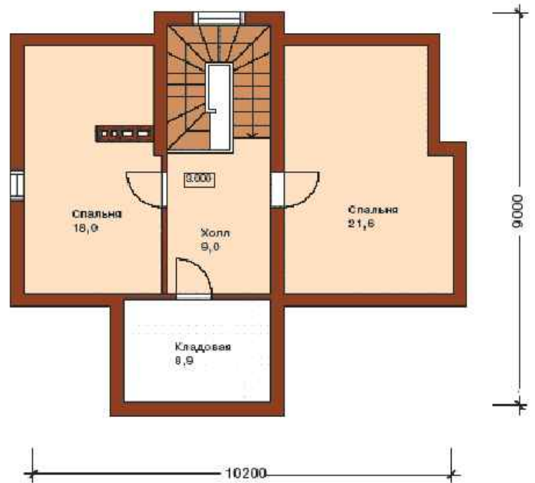
План мансардного этажа
