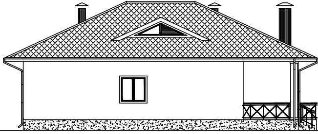
Фасад в осях В-А.
