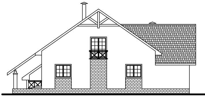
Фасад в осях 5-1.
