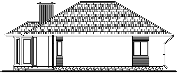
Фасад в осях 5-1.
