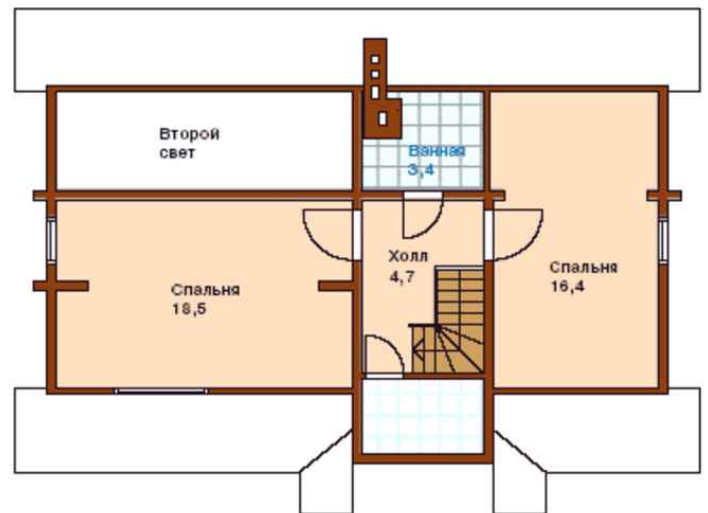
План мансардного этажа
