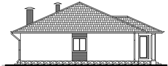
Фасад в осях В-А.
