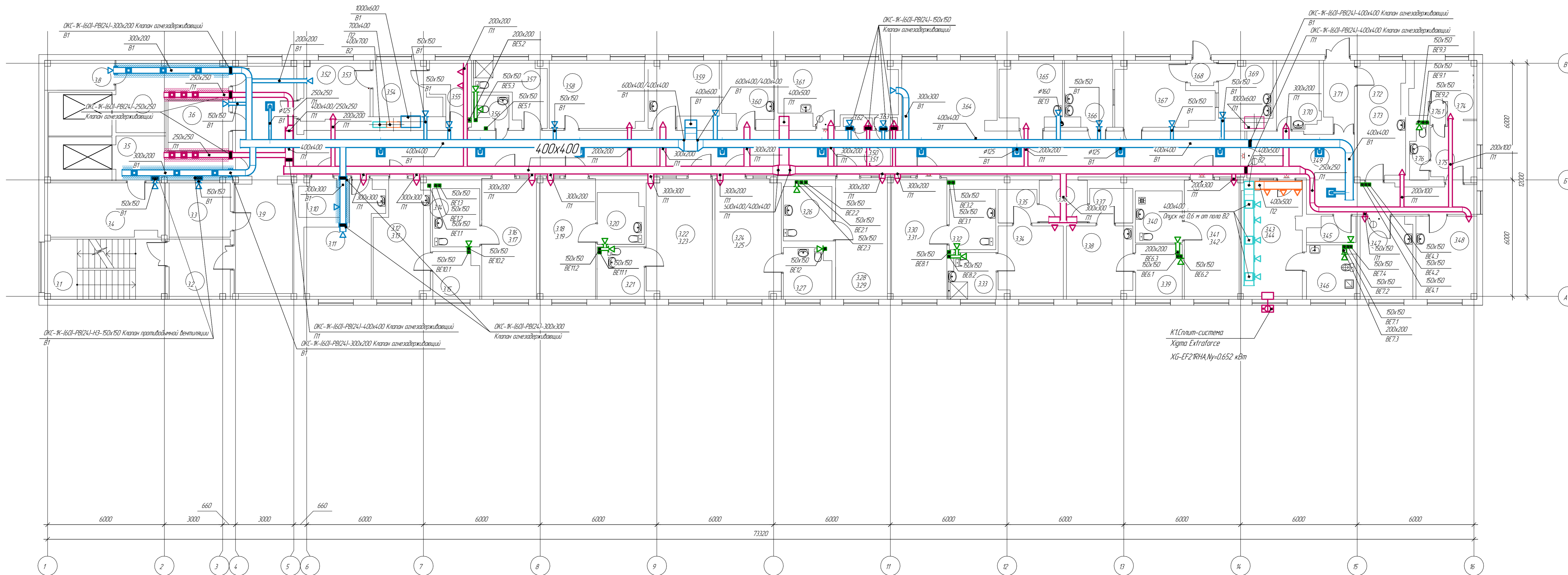
Экспликация помещений 3 этажа 1-го корпуса
