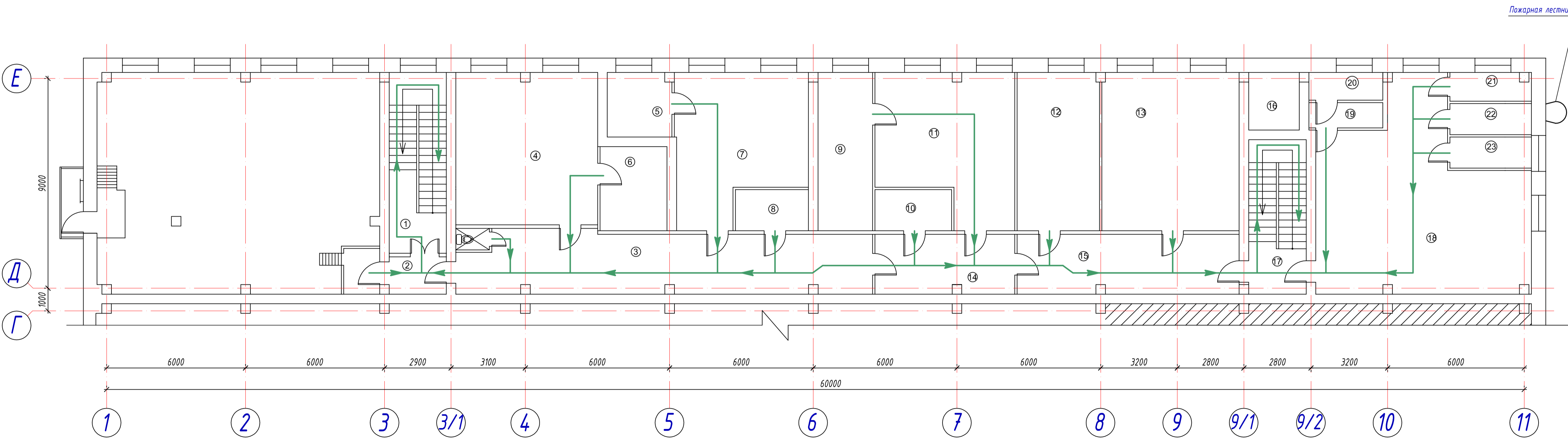
План 3 этажа на отметке +7,200
