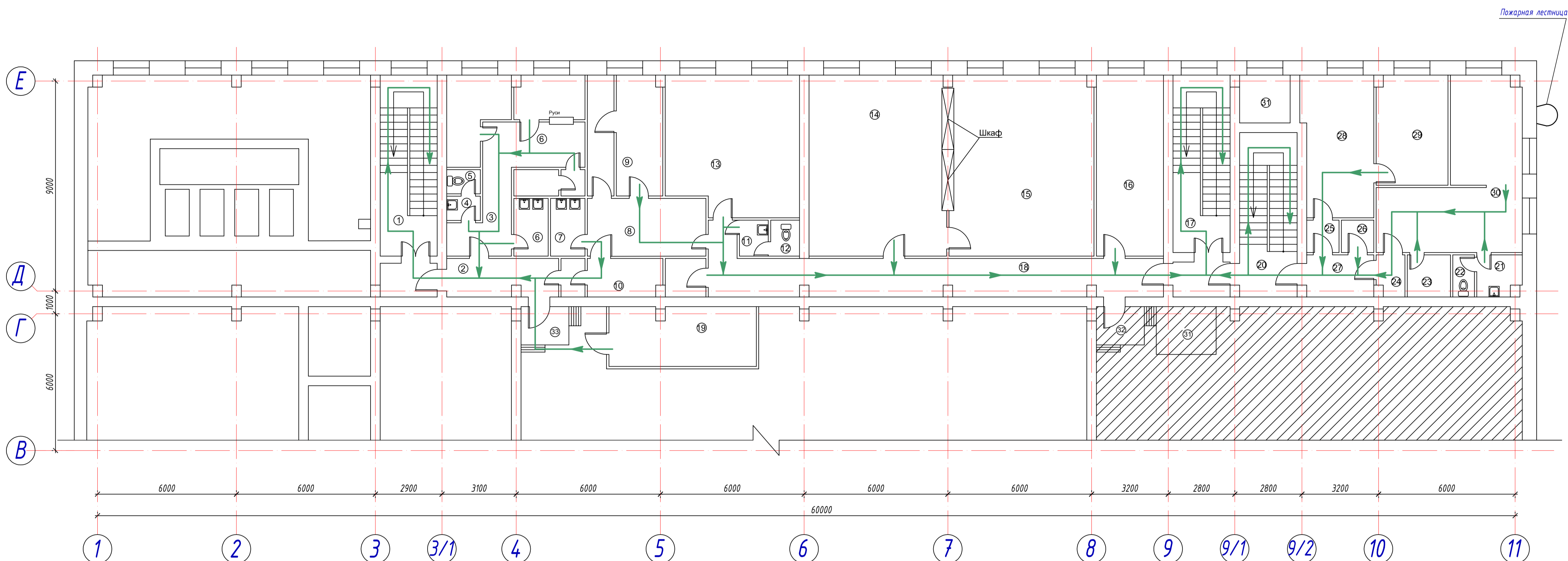
План 2 этажа на отметке +3,600
