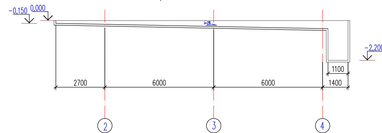
Разрез 1-1
