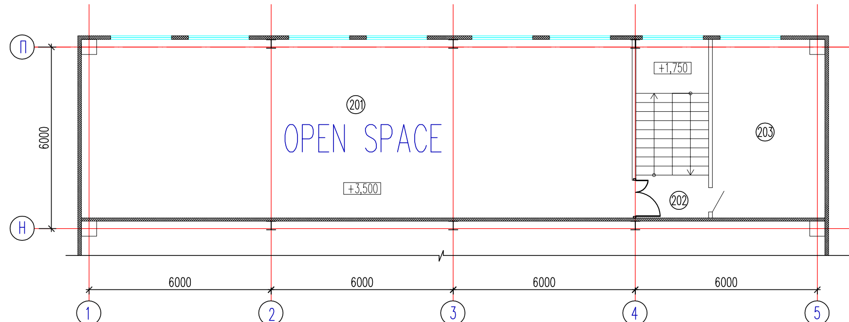
План на отм. +3,500
