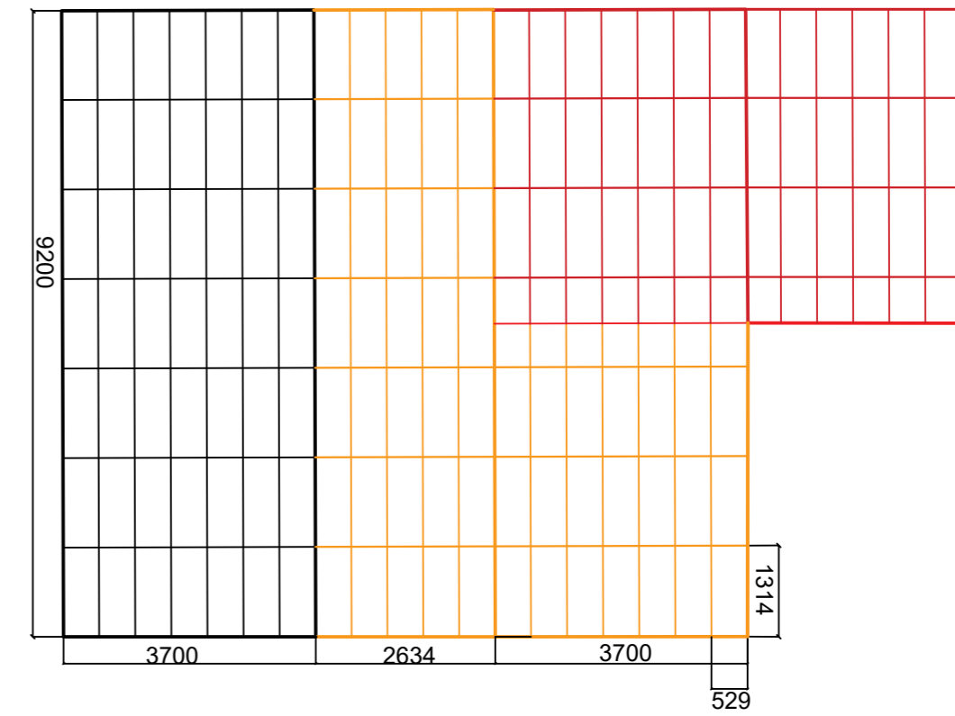
Схема развёртки стропильного скелета
