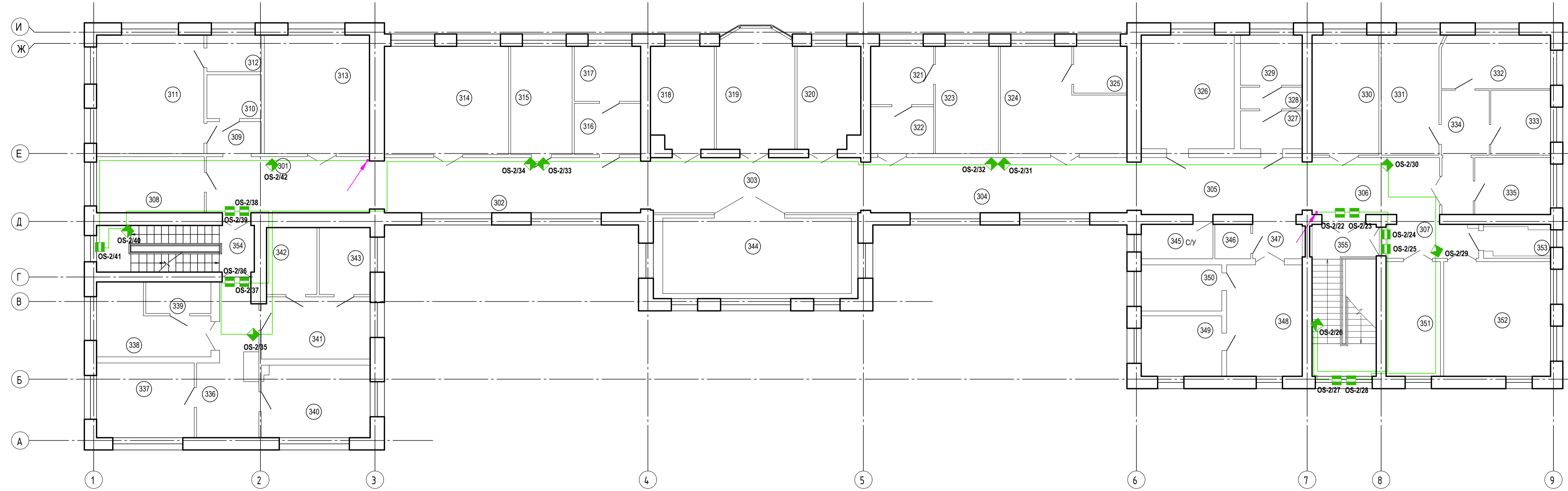
План 3-его этажа
