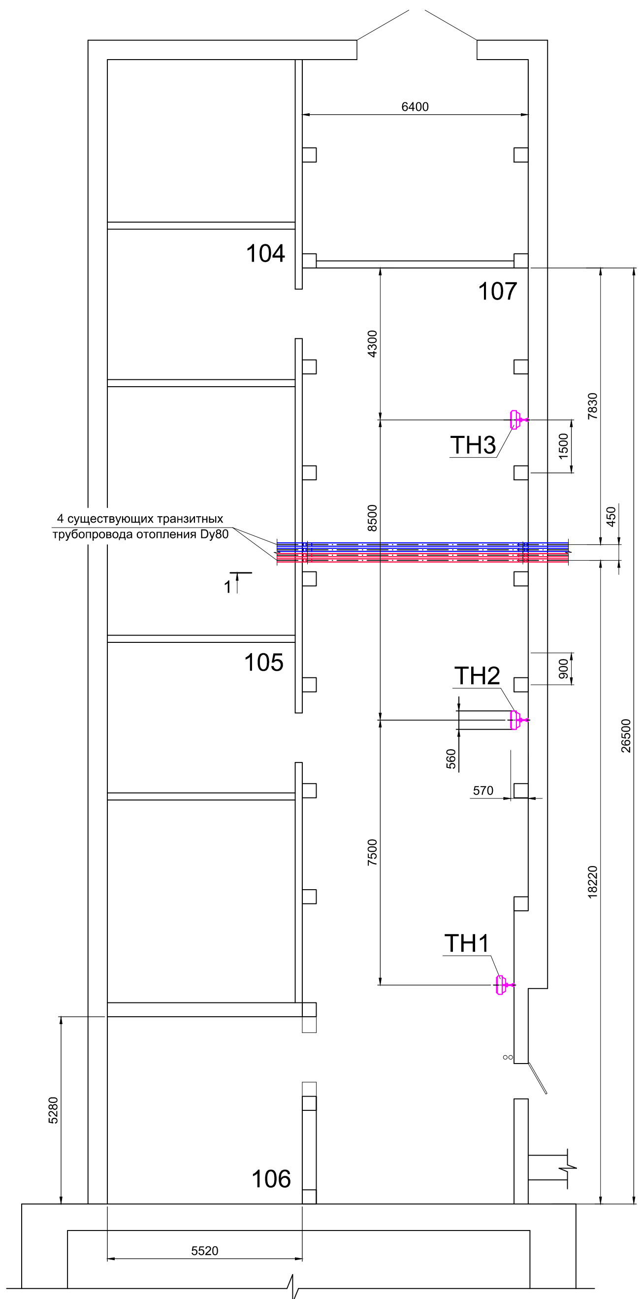
План (1:100)
