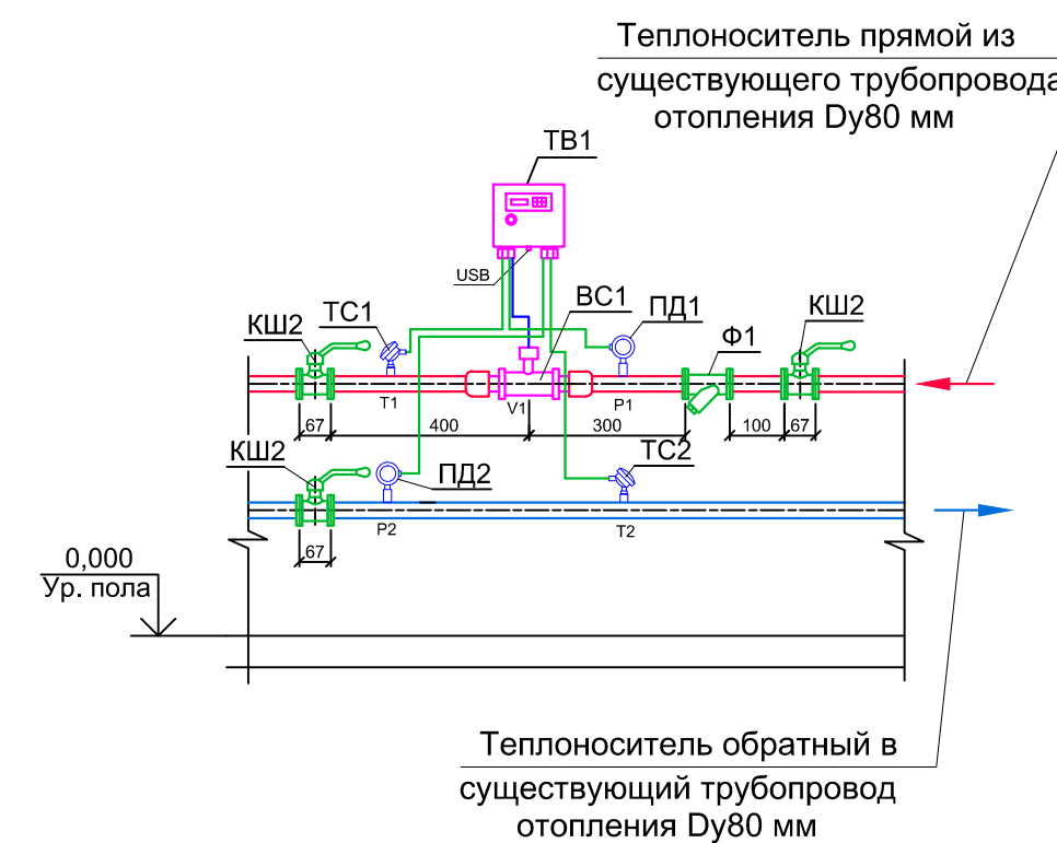
Узел установки тепловычислителя*
