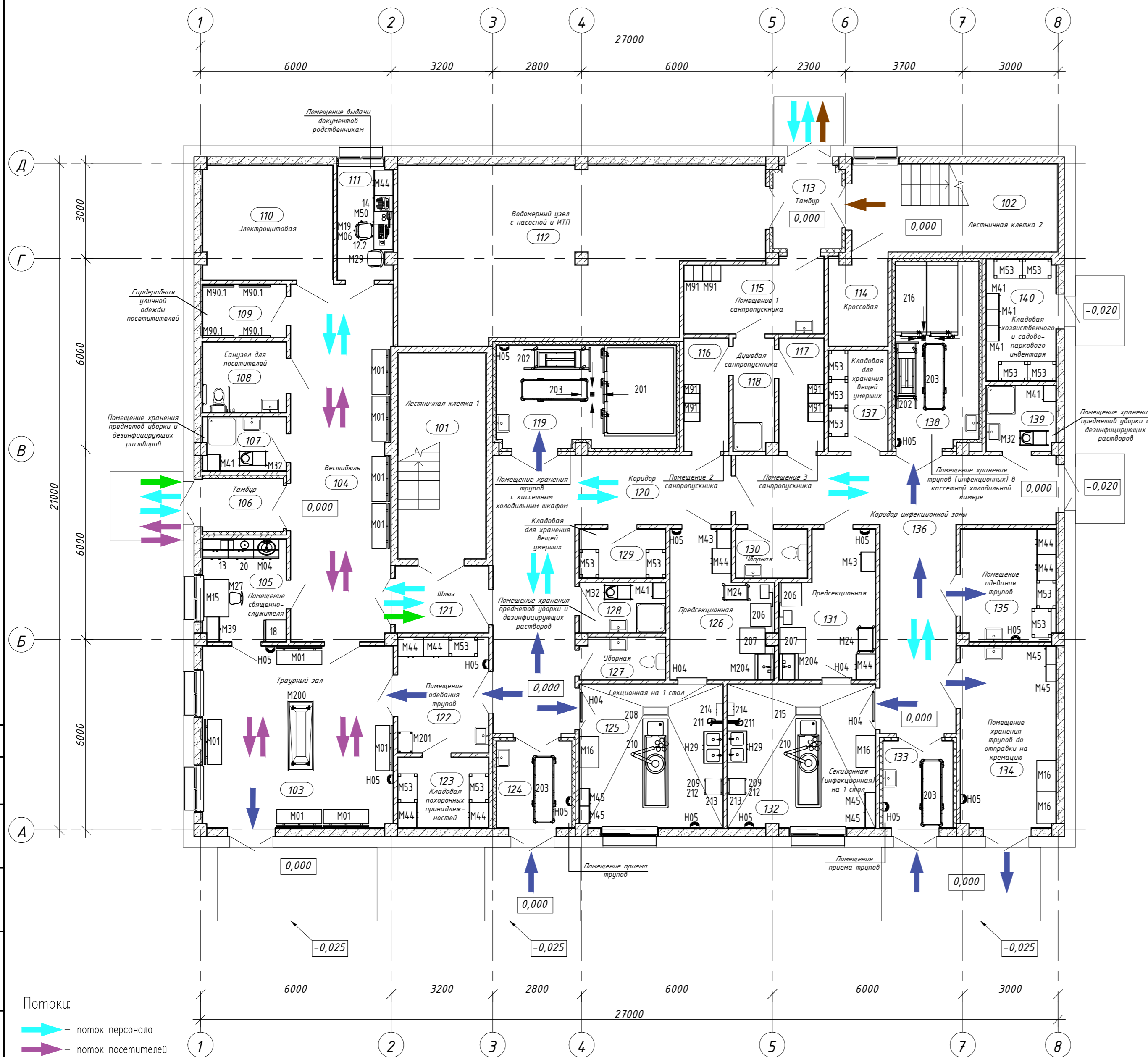
План 1-го этажа
