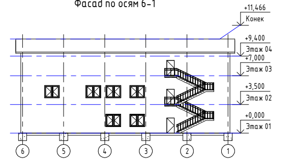
Фасад по осям 6-1
