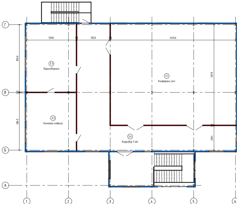
План на отметке +7,000
