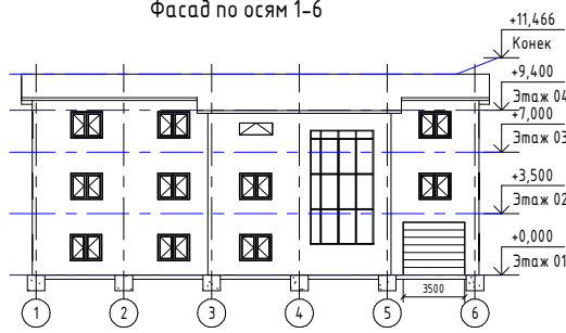
Фасад по осям 1-6
