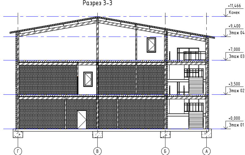
Разрез 3-3
