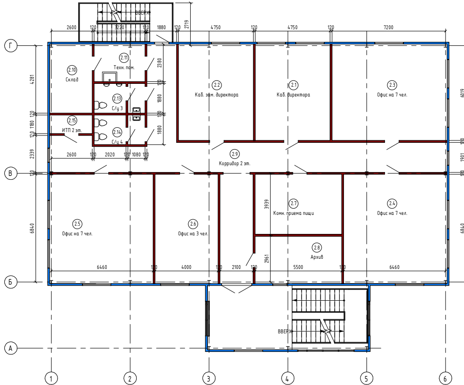
План на отметке +3,500
