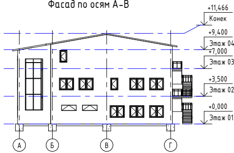
Фасад по осям А-В
